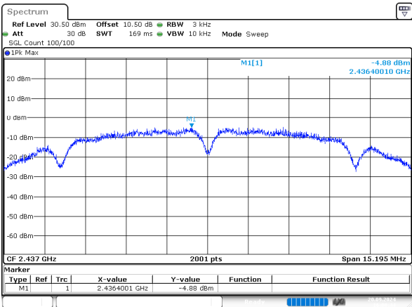
b_2437MHz_Chain 1
