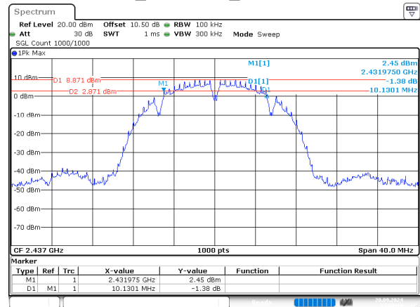
b_2437MHz_Chain 0
