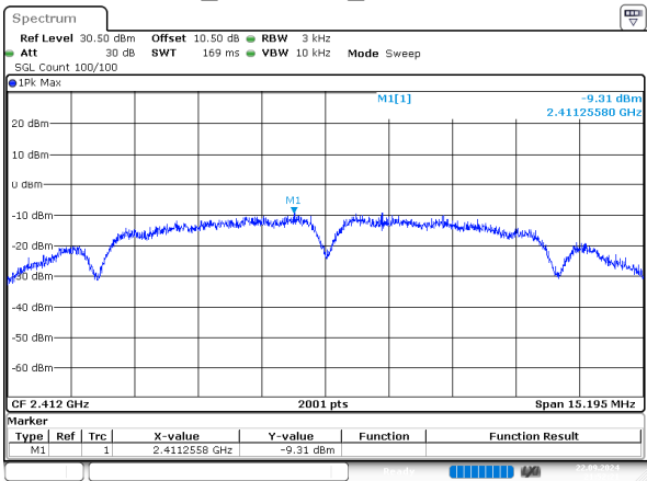
b_2412MHz_Chain 0
