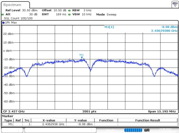
b_2437MHz_Chain 0
