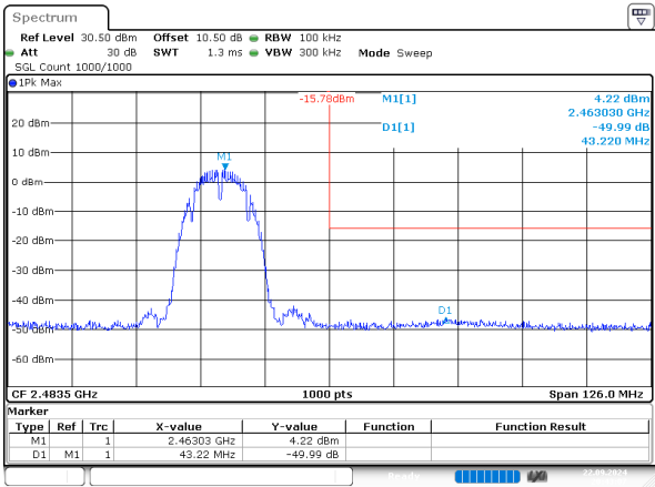
b_2462MHz_Chain 0
