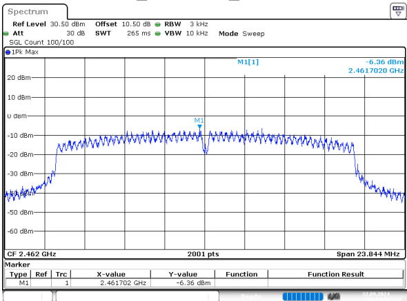
n20_2462MHz_Chain 0
