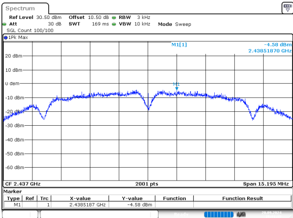
b_2437MHz_Chain 0
