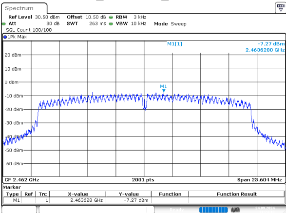
n20_2462MHz_Chain 1
