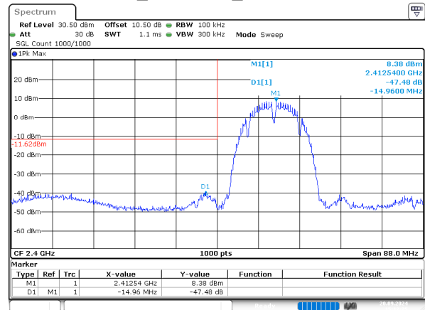
b_2412MHz_Chain 1
