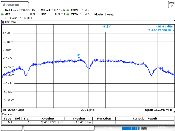
b_2437MHz_Chain 1
