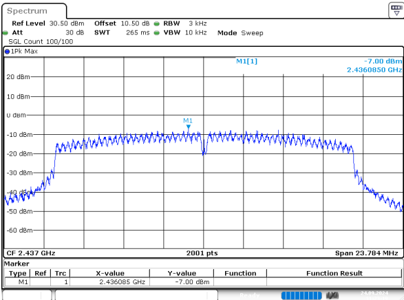
n20_2437MHz_Chain 1
