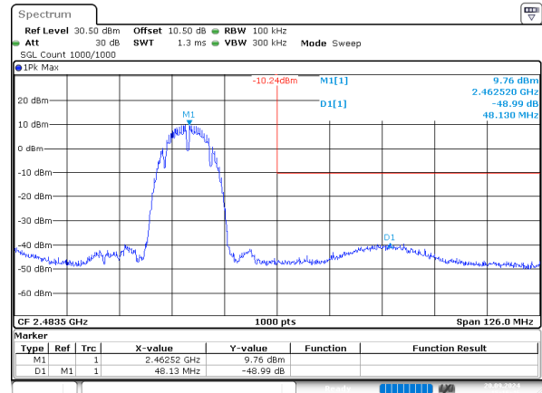
b_2462MHz_Chain 1
