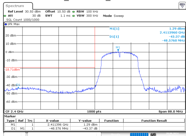
n20_2412MHz_Chain 1
