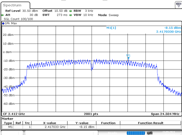
n20_2412MHz_Chain 1
