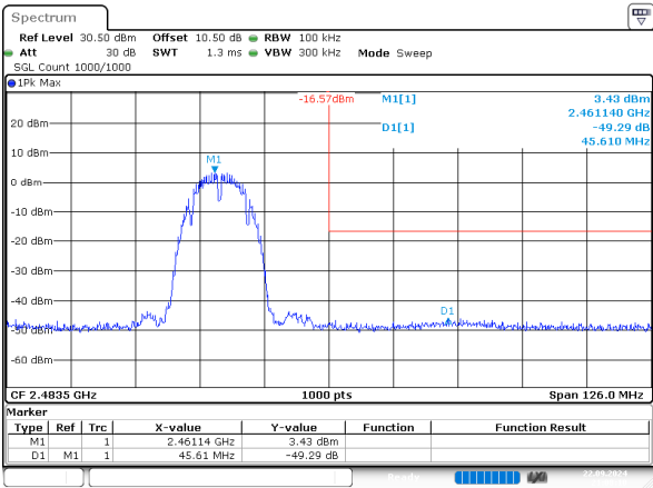
b_2462MHz_Chain 1
