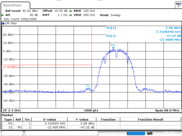
b_2412MHz_Chain 1
