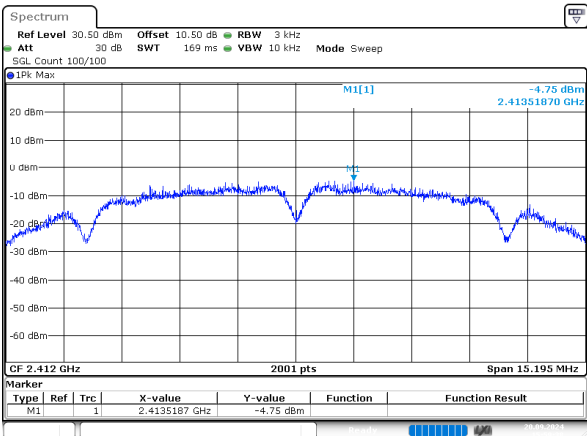
b_2412MHz_Chain 1
