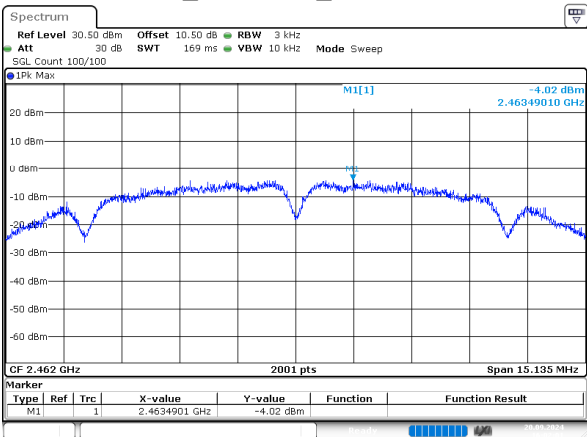
b_2462MHz_Chain 1
