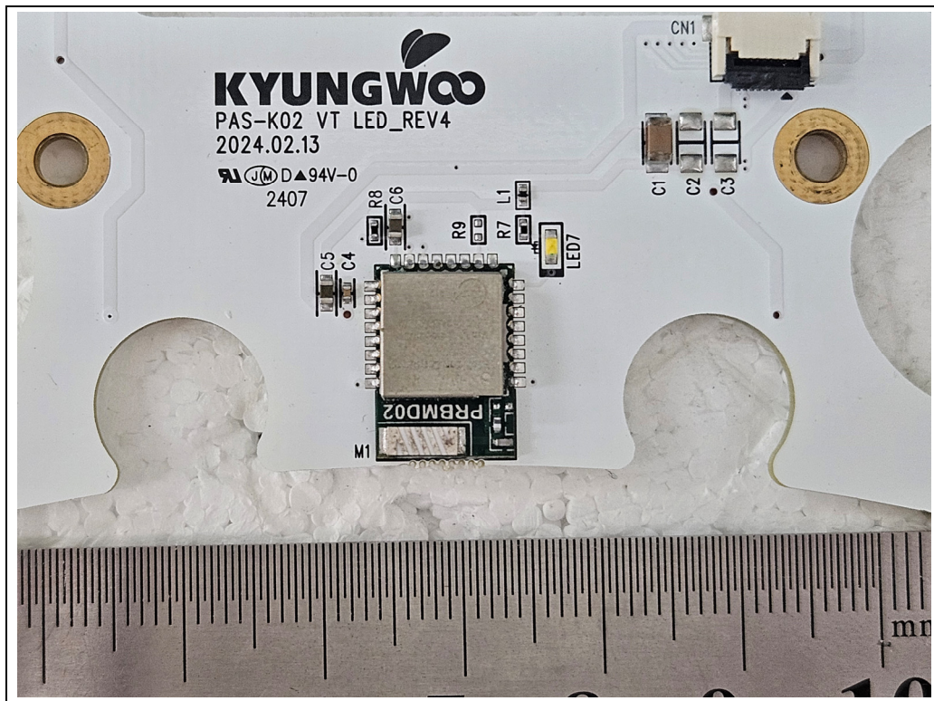
&lt;BLE Module&gt;
