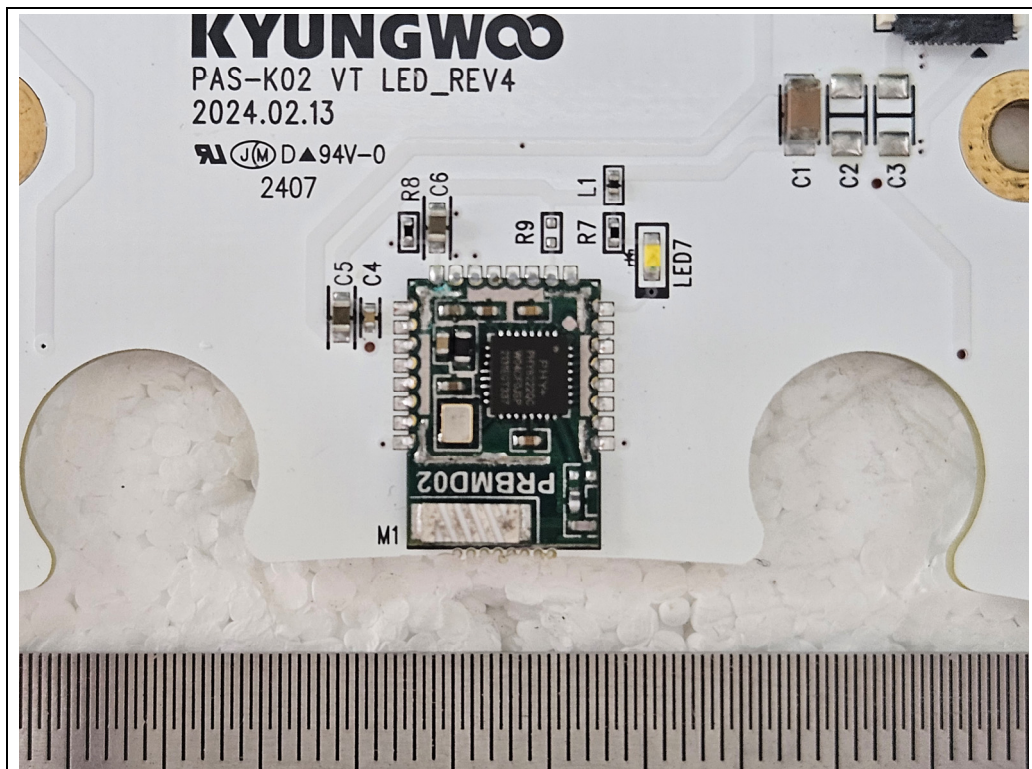
&lt;BLE Module&gt;
