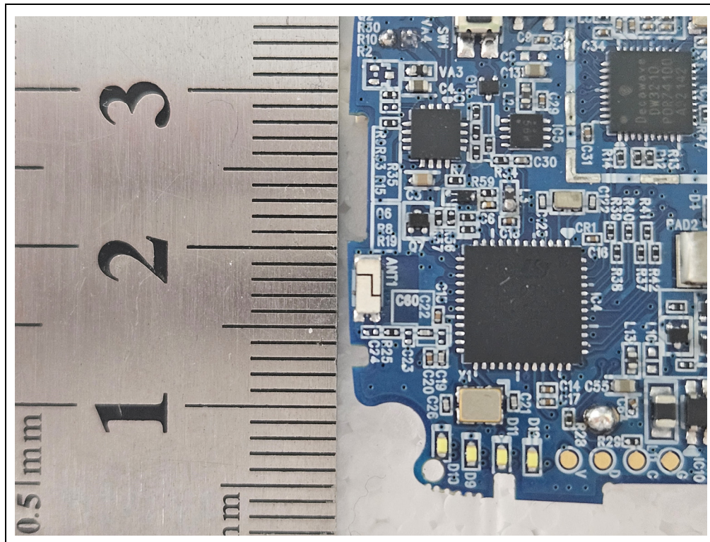
Antenna
