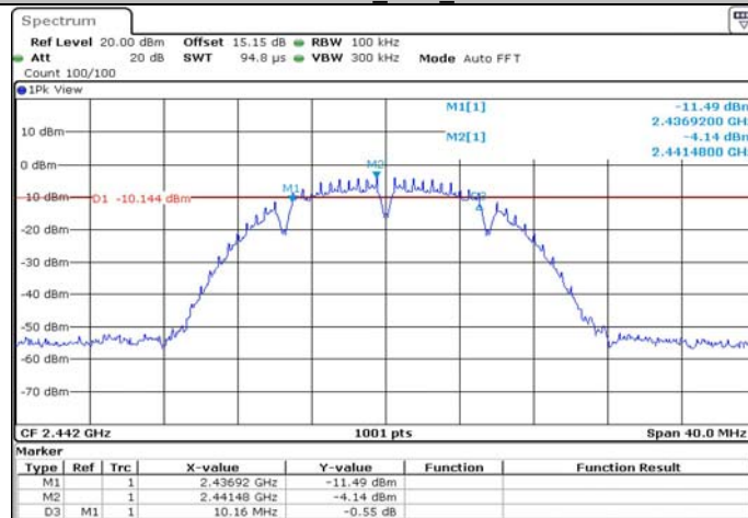
11BMIMO_Ant1_2442
