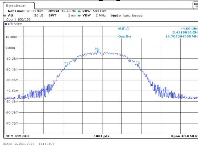
11BMIMO_Ant2_2412
