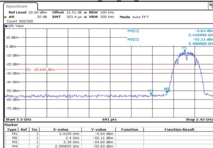
11BMIMO_Ant2_Low_2412
