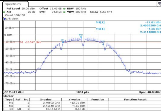
11BMIMO_Ant1_2412
