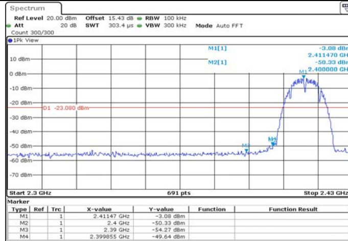
11BMIMO_Ant1_Low_2412
