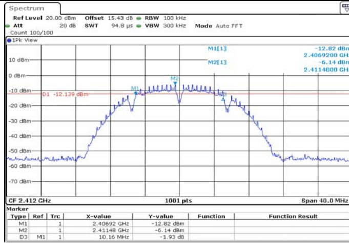
11B-CDD_Ant1_2412
