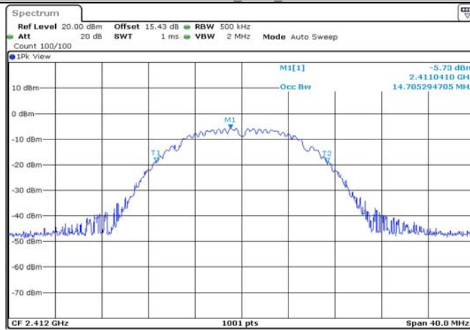
11B-CDD_Ant1_2412
