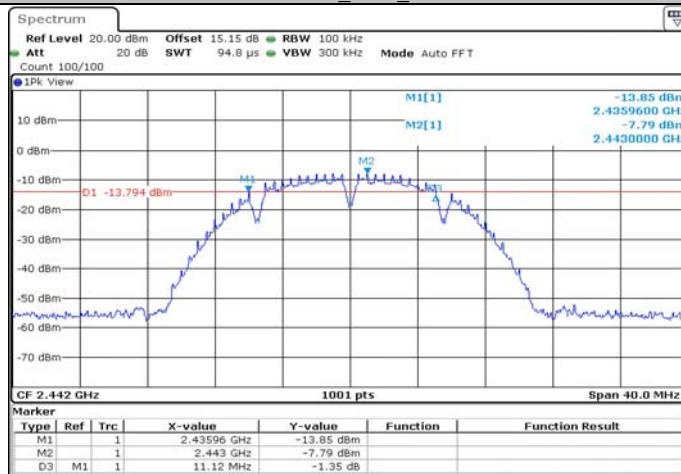
11B-CDD_Ant1_2442
