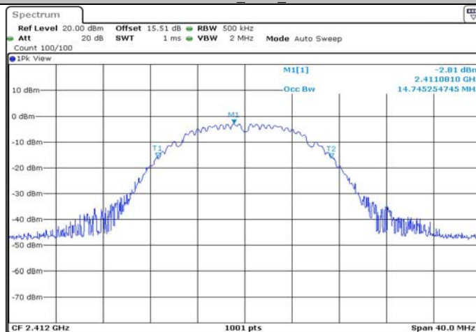
11B-CDD_Ant2_2412
