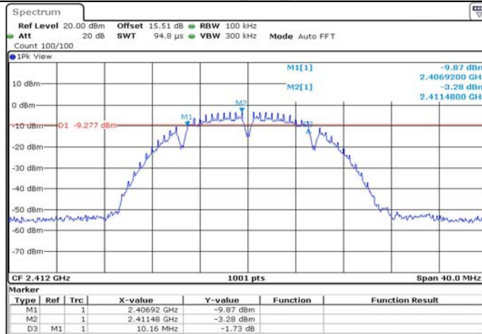
11B-CDD_Ant2_2412
