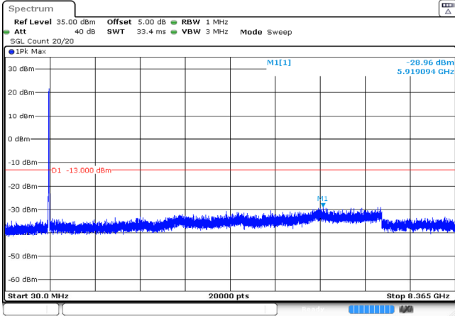
10MHz_Middle_QPSK_50@0 -28.96dBm
