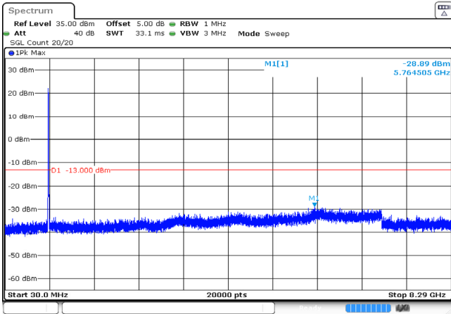
10MHz_Low_QPSK_50@0 -28.89dBm
