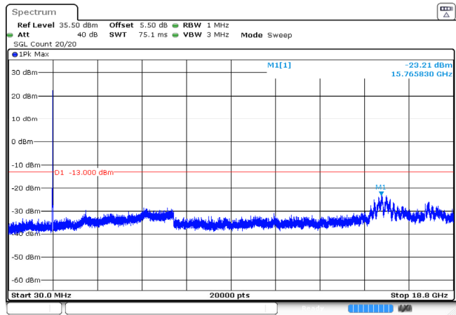
10MHz_Middle_QPSK_50@0 -23.21dBm
