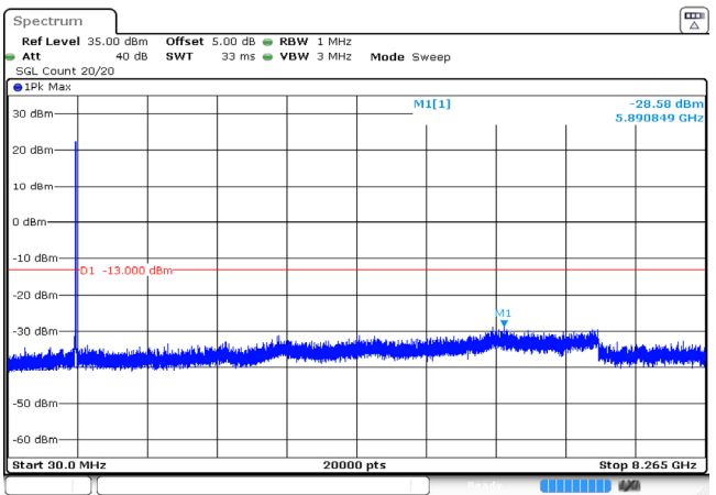
5MHz_Low_QPSK_25@0 -28.58dBm
