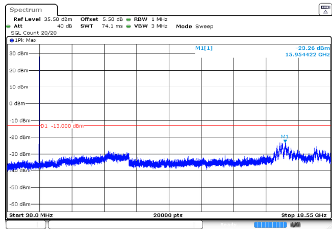
10MHz_Low_QPSK_1@0 -23.26dBm
