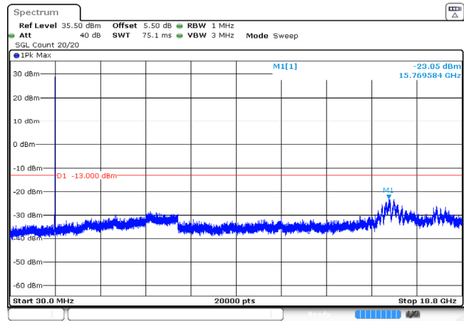
10MHz_Middle_QPSK_1@0 -23.05dBm
