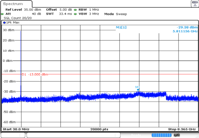
10MHz_Middle_QPSK_1@0 -29.38dBm
