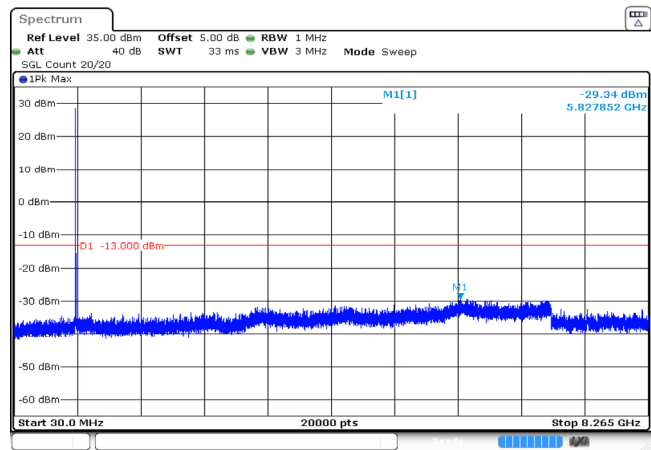
5MHz_Low_QPSK_1@0 -29.34dBm
