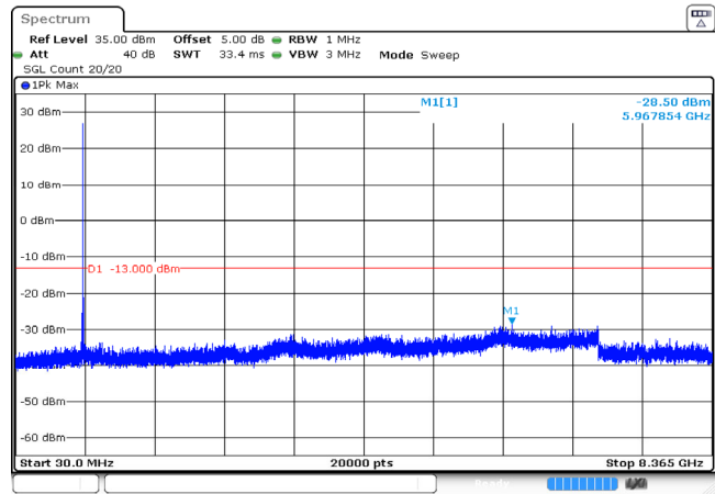
5MHz_Middle_QPSK_1@0 -28.50dBm
