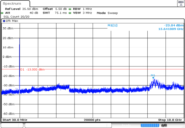
20MHz_Middle_QPSK_100@0 -23.04dBm
