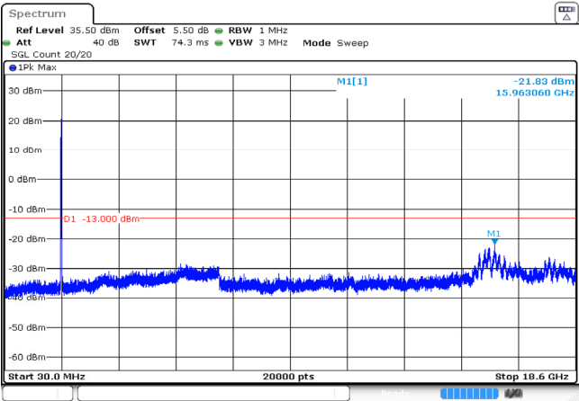
20MHz_Low_QPSK_100@0 -21.83dBm
