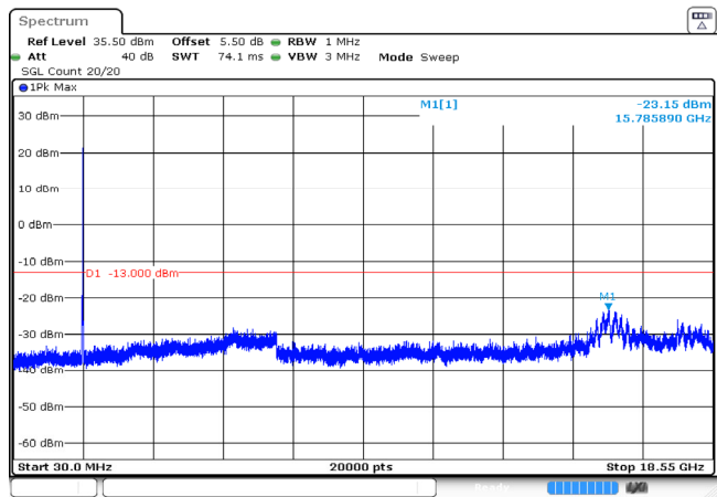
10MHz_Low_QPSK_50@0 -23.15dBm
