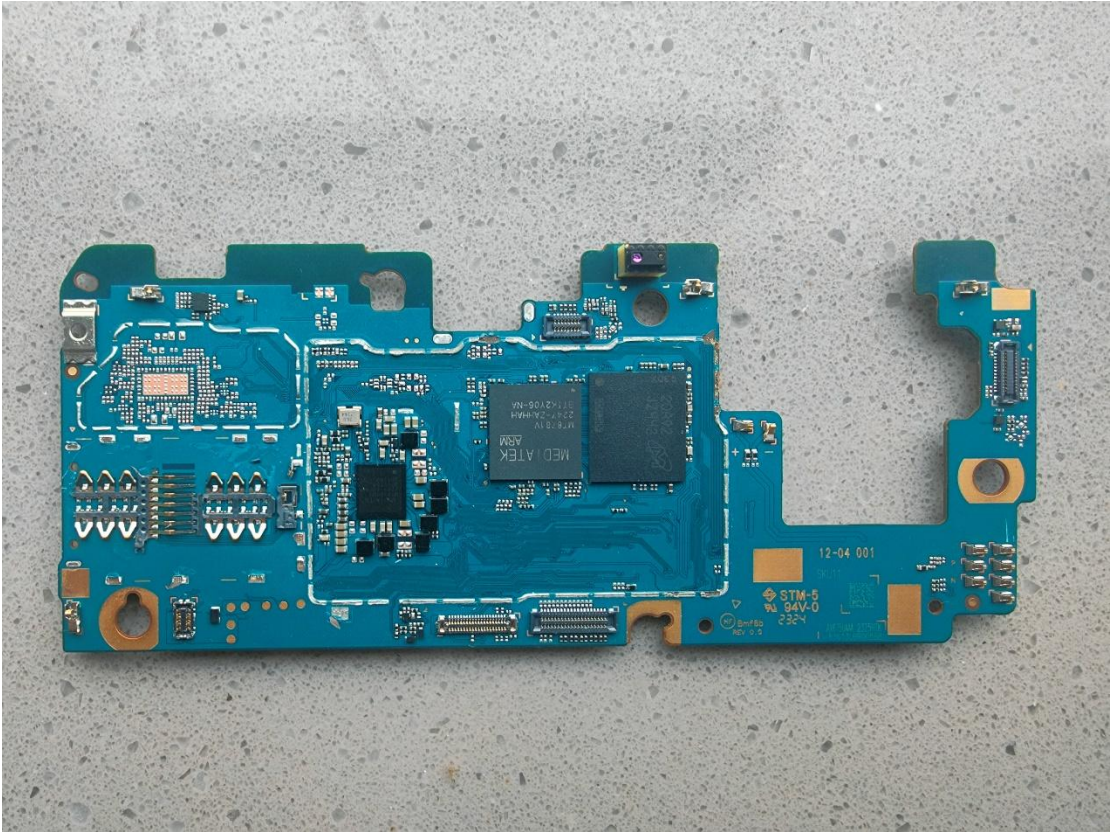
PCB10
