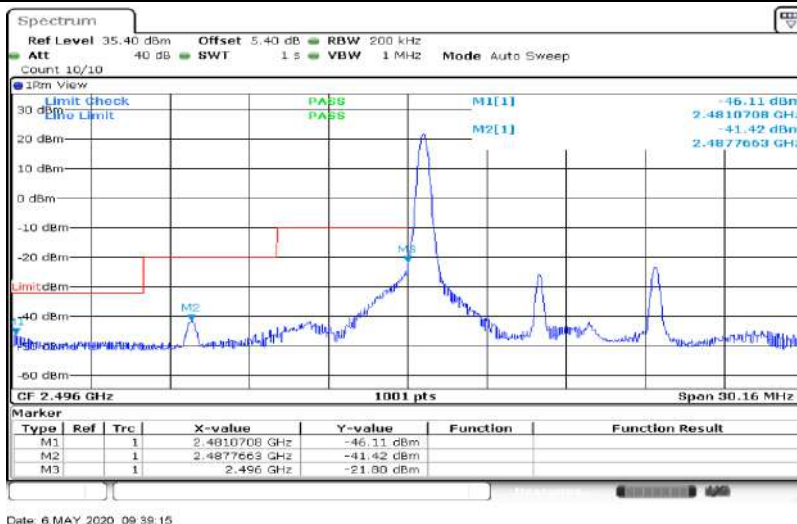
Band41-10MHz-QPSK-39700-50RB#0
