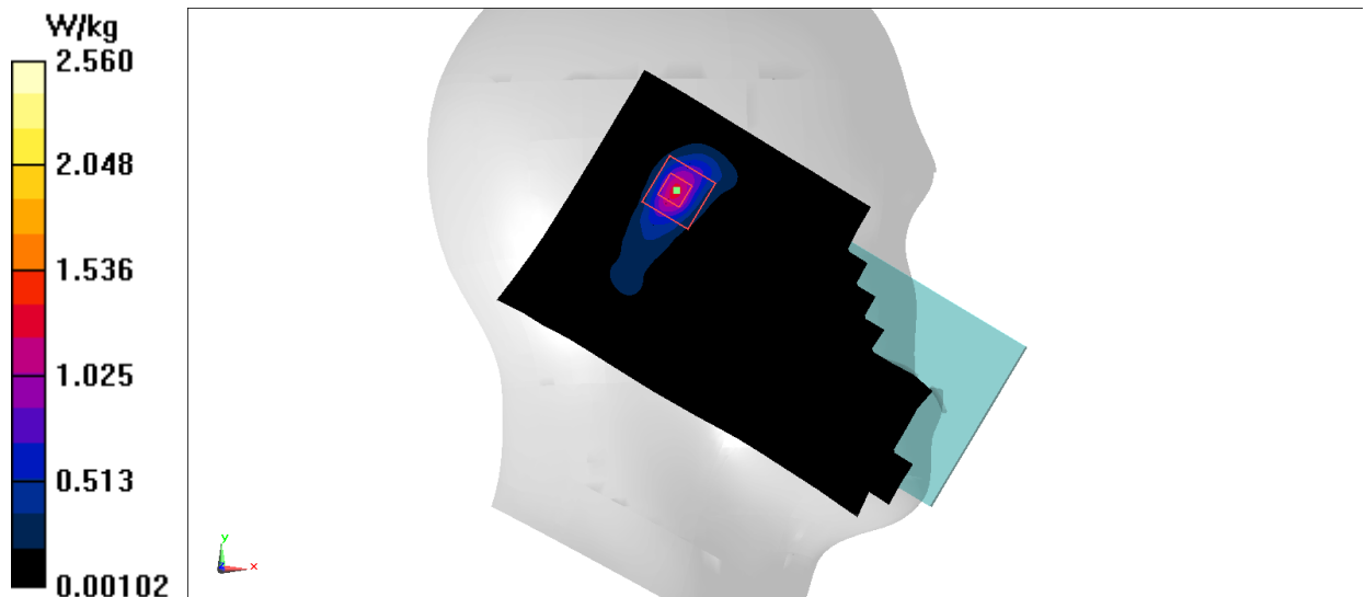
Fig.19 5GHz
