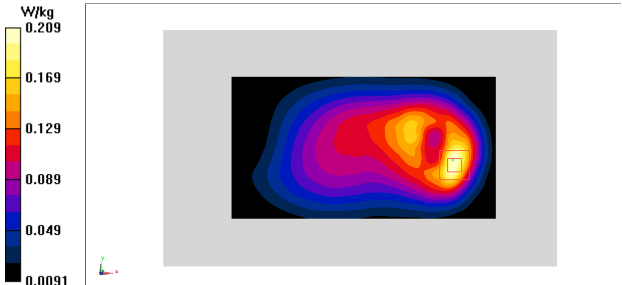
Fig.12 LTE Band5
