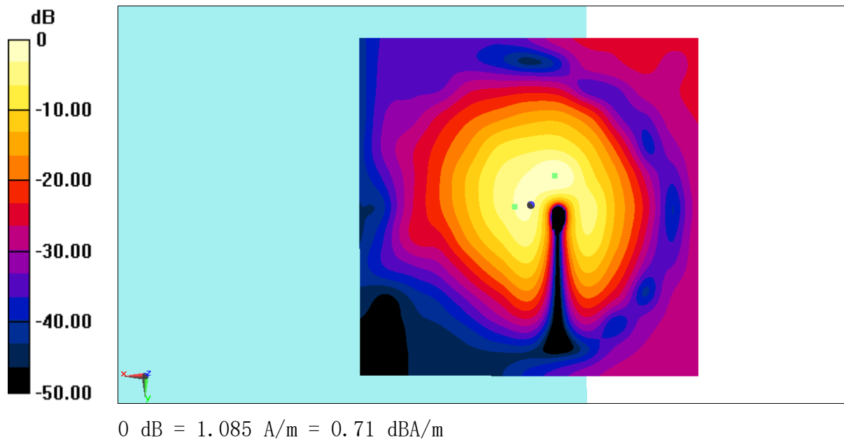
Fig B.12 T-Coil WCDMA 1900 -OTT
