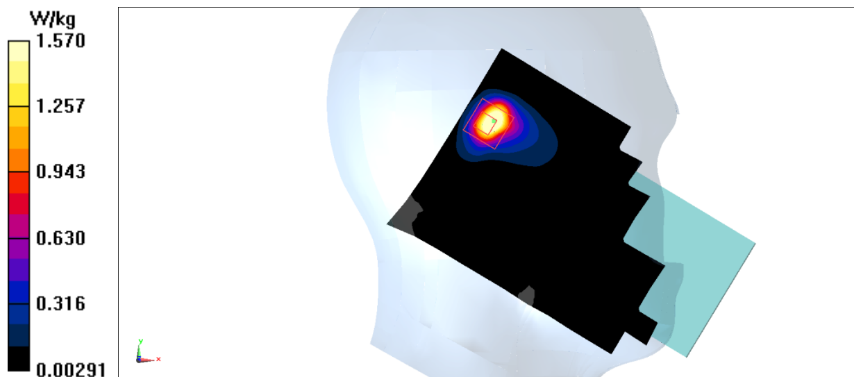
Fig.19 2450 MHz
