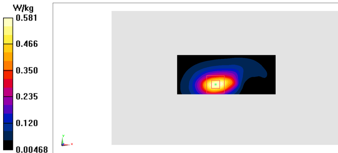
Fig.10 LTE Band7
