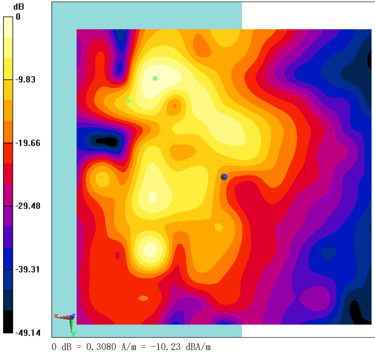
Fig B.19 T-Coil WiFi-2. 4G
