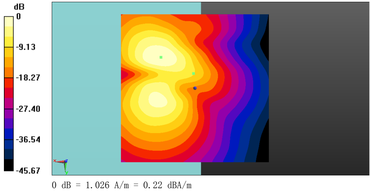
Fig B.15 T-Coil LTE B5
