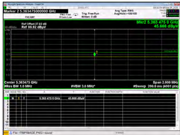
U-NII-2A 11ax80 CH58 AV
