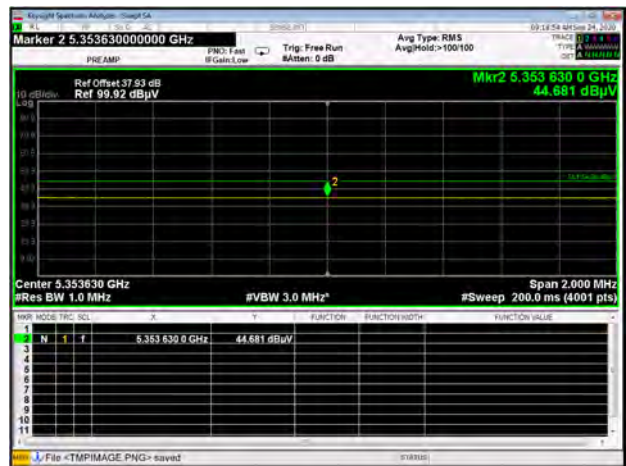
U-NII-2A 11ax20 CH64 AV
