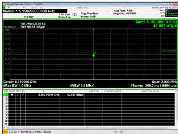
U-NII-1 11ax40 CH38 AV
