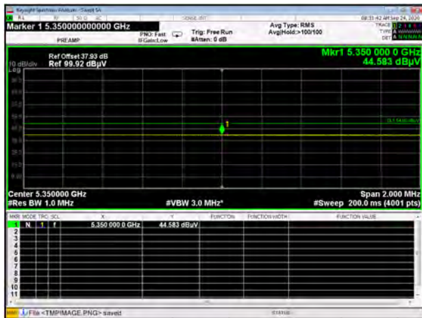
U-NII-2A 11a CH64 AV
