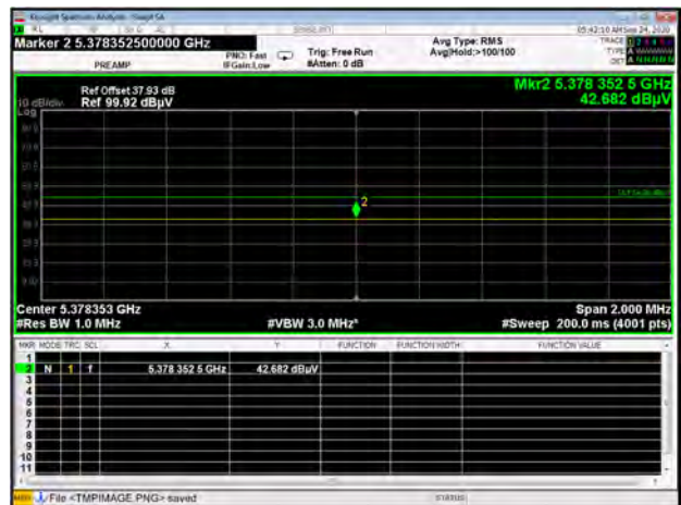
U-NII-1 11ac40 CH46 AV
