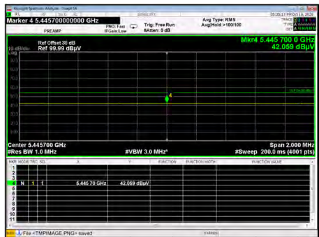
U-NII-2C 11ac80 CH138 AV
