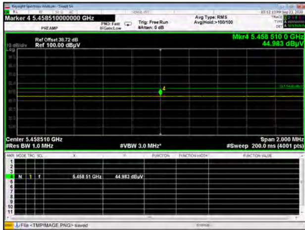
U-NII-2C 11ac160 CH114 AV
