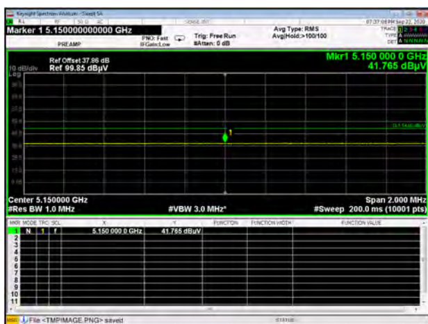
U-NII-1 11ax20 CH36 AV
