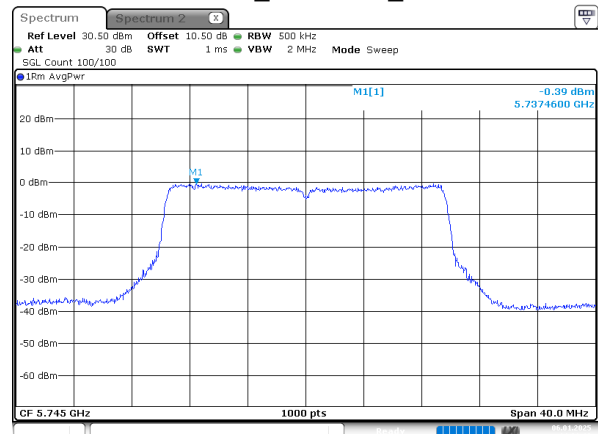
802.11be20_5745MHz_Chain 1
