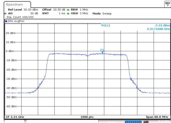
802.11be40_5310MHz_Chain 1
