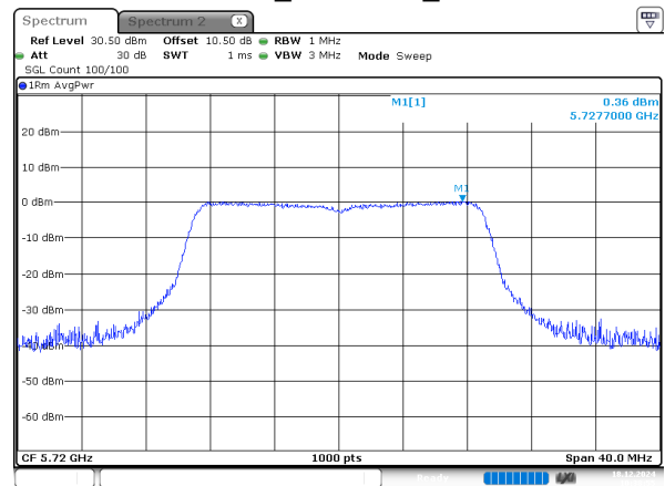
802.11n20_5720MHz_Chain 1
