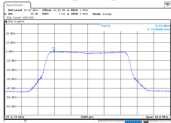
802.11be20_5720MHz_Chain 3
