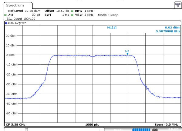
802.11be20_5580MHz_Chain 2
