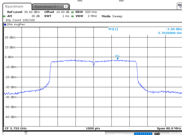
802.11be40_5755MHz_Chain 1
