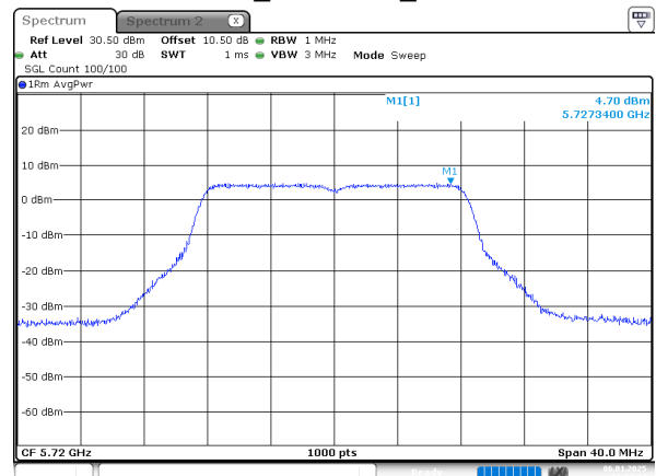
802.11a_5720MHz_Chain 2
