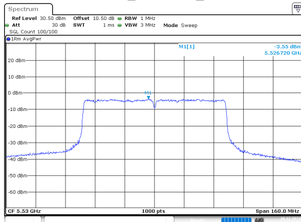
802.11ac80_5530MHz_Chain 2
