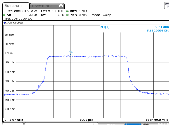
802.11be40_5670MHz_Chain 1
