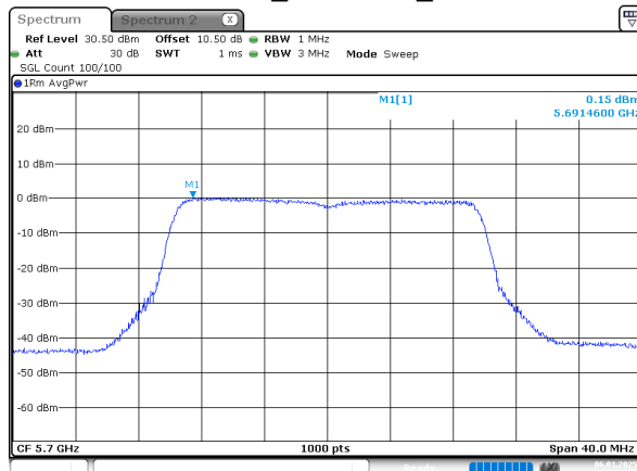
802.11be20_5700MHz_Chain 0
