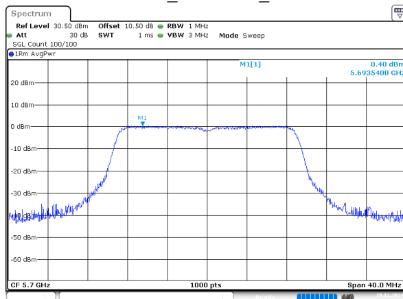
802.11n20_5700MHz_Chain 2
