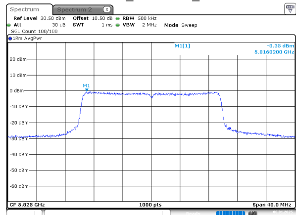
802.11be20_5825MHz_Chain 1
