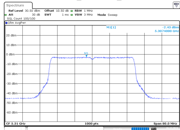
802.11be40_5310MHz_Chain 2
