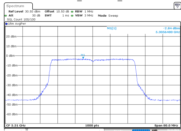
802.11be40_5310MHz_Chain 3
