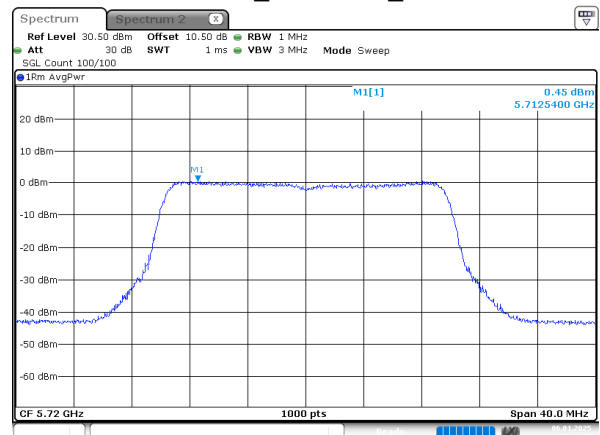
802.11be20_5720MHz_Chain 1
