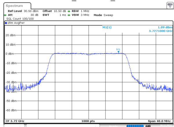
802.11n20_5720MHz_Chain 2
