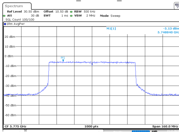
802.11be80_5775MHz_Chain 2
