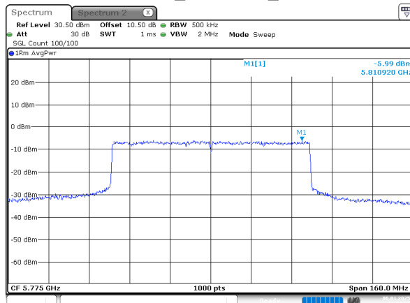
802.11be80_5775MHz_Chain 0
