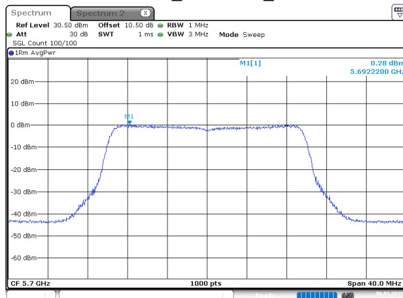
802.11be20_5700MHz_Chain 1
