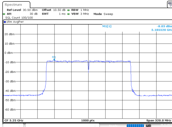
802.11be160_5250MHz_Chain 2
