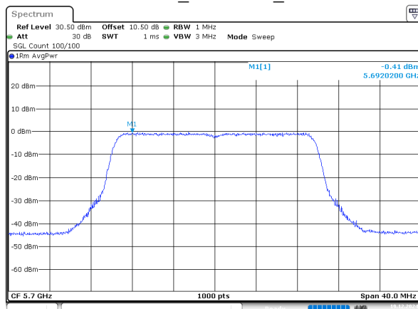
802.11be20_5700MHz_Chain 2
