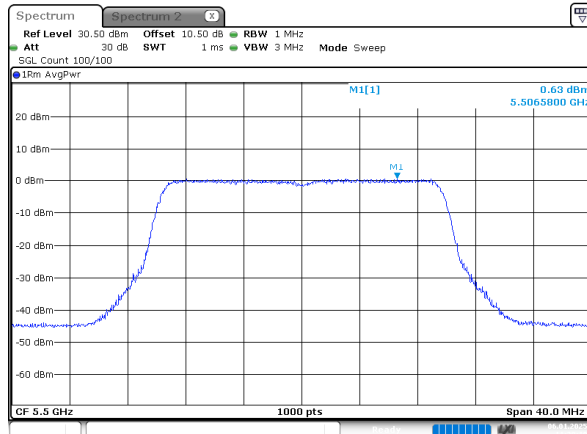
802.11be20_5500MHz_Chain 0
