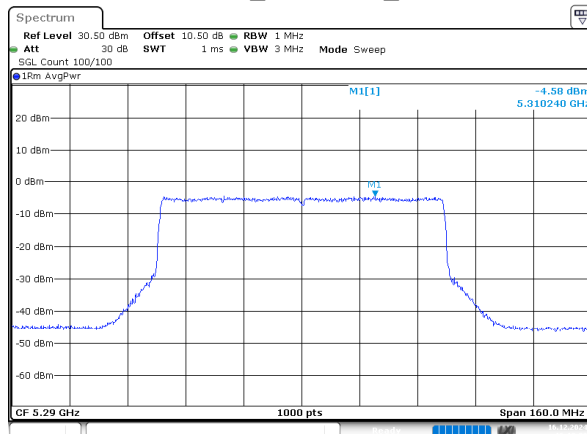
802.11be80_5290MHz_Chain 2
