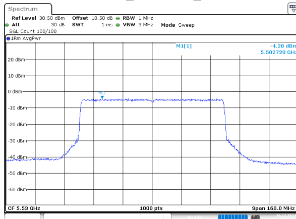
802.11be80_5530MHz_Chain 2
