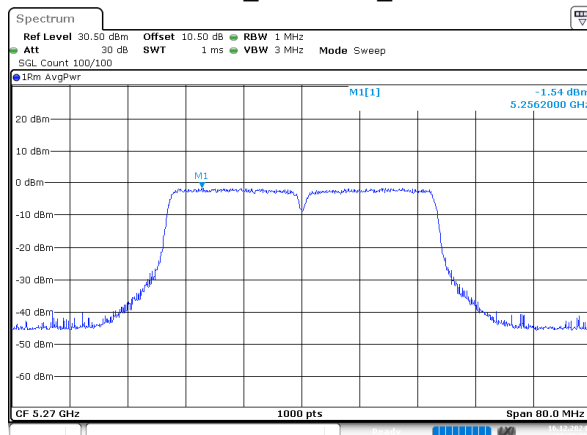
802.11n40_5270MHz_Chain 3
