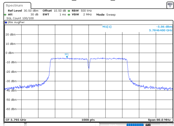
802.11n40_5795MHz_Chain 3
