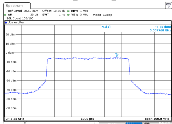
802.11be80_5530MHz_Chain 3
