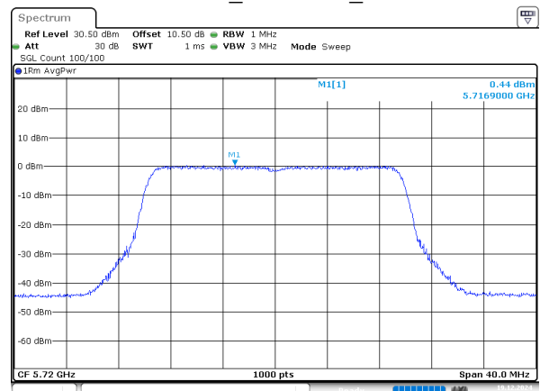
802.11be20_5720MHz_Chain 2
