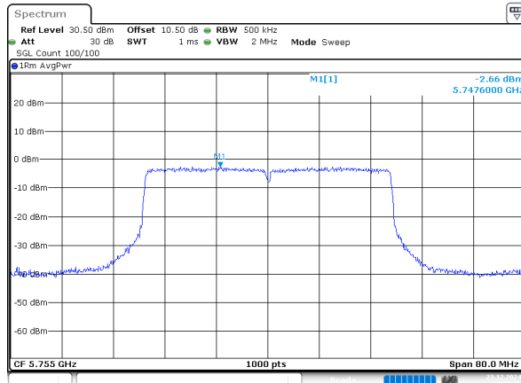
802.11be40_5755MHz_Chain 3
