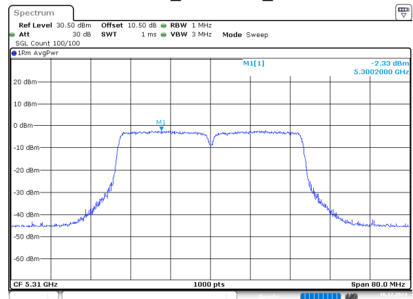
802.11n40_5310MHz_Chain 3
