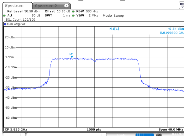
802.11be20_5825MHz_Chain 0
