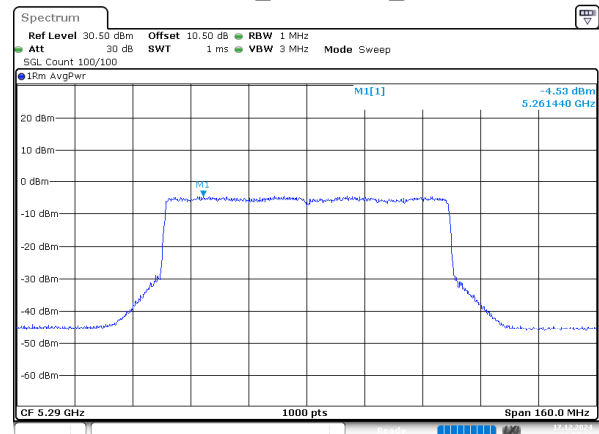
802.11be80_5290MHz_Chain 3
