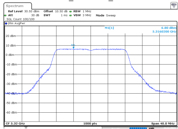
802.11a_5320MHz_Chain 3
