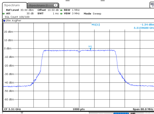
802.11be40_5510MHz_Chain 0
