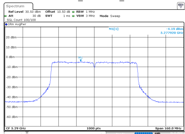
802.11ac80_5290MHz_Chain 3
