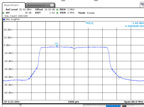
802.11be40_5510MHz_Chain 1
