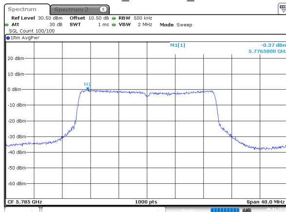
802.11be20_5785MHz_Chain 1
