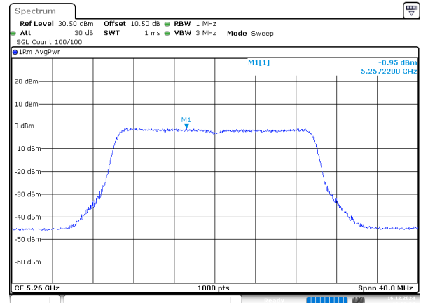
802.11be20_5260MHz_Chain 3
