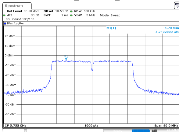
802.11n40_5755MHz_Chain 3
