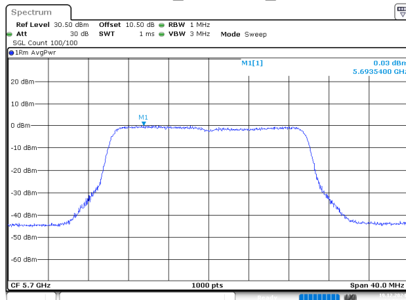
802.11be20_5700MHz_Chain 3
