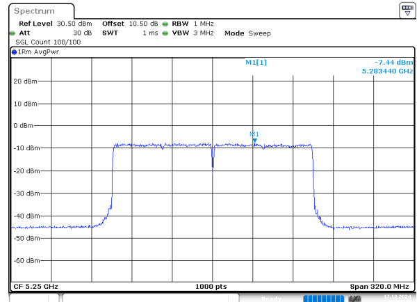
802.11be160_5250MHz_Chain 3
