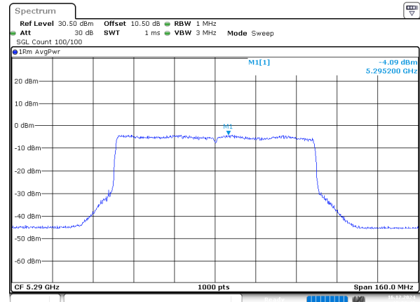
802.11be80_5290MHz_Chain 1
