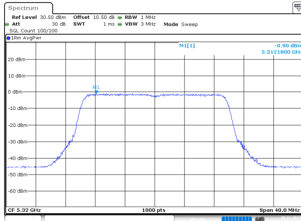
802.11be20_5320MHz_Chain 2
