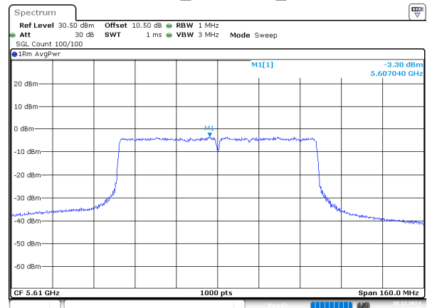
802.11ac80_5610MHz_Chain 2
