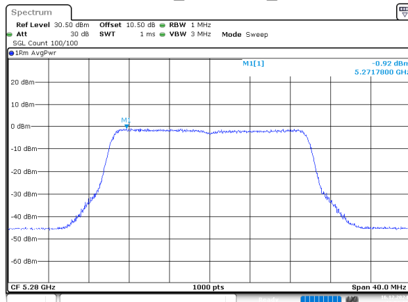
802.11be20_5280MHz_Chain 3
