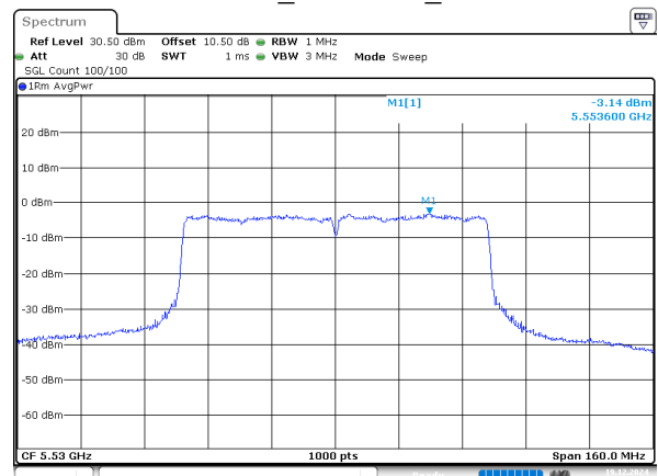
802.11ac80_5530MHz_Chain 3
