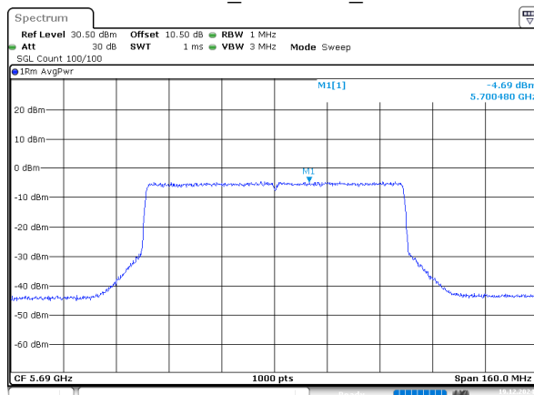
802.11be80_5690MHz_Chain 2
