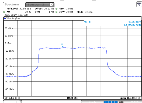
802.11be80_5690MHz_Chain 1
