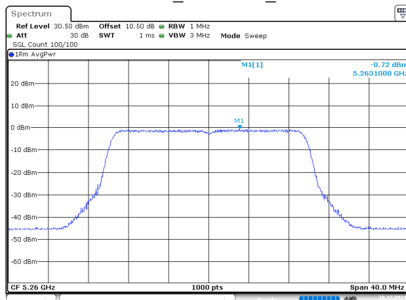
802.11be20_5260MHz_Chain 0
