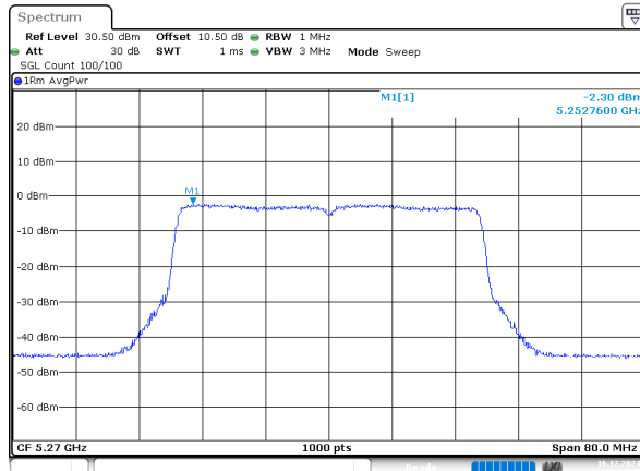
802.11be40_5270MHz_Chain 1
