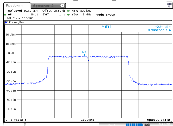
802.11be40_5795MHz_Chain 0
