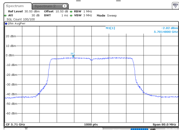
802.11be40_5710MHz_Chain 1
