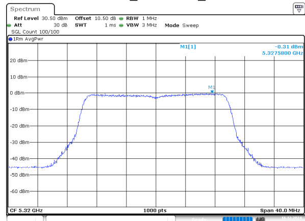
802.11be20_5320MHz_Chain 1
