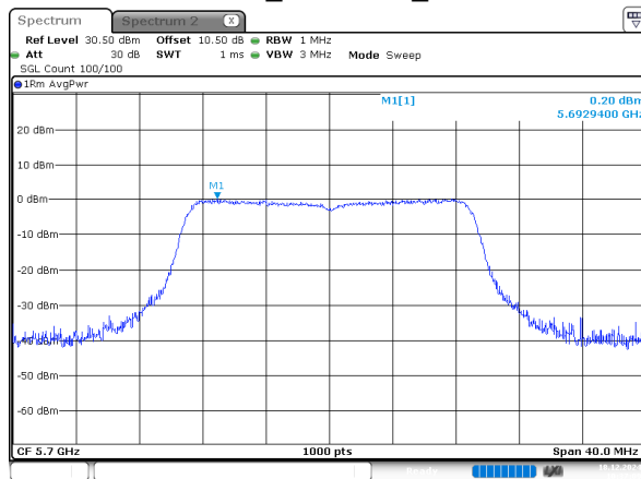
802.11n20_5700MHz_Chain 1
