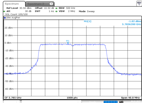
802.11be20_5785MHz_Chain 0
