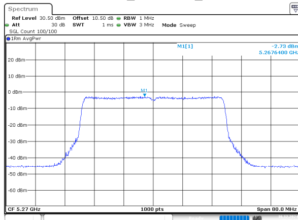
802.11be40_5270MHz_Chain 2
