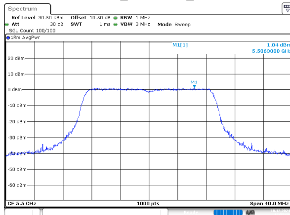
802.11n20_5500MHz_Chain 2
