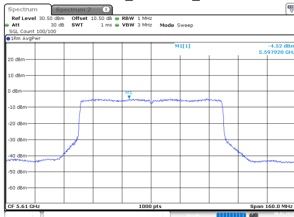
802.11be80_5610MHz_Chain 1
