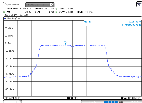
802.11be40_5710MHz_Chain 0
