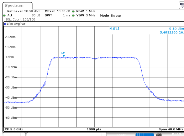
802.11be20_5500MHz_Chain 2
