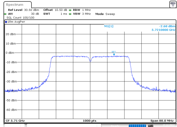
802.11n40_5710MHz_Chain 0
