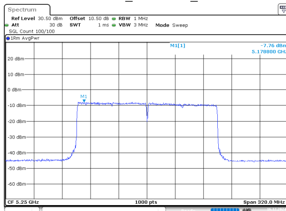
802.11be160_5250MHz_Chain 0
