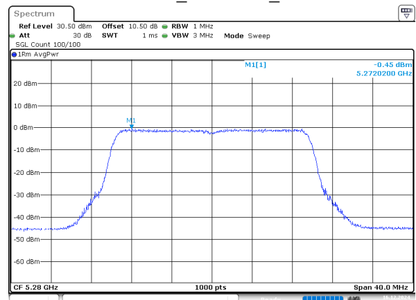
802.11be20_5280MHz_Chain 0
