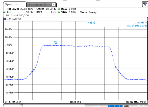
802.11be20_5720MHz_Chain 0
