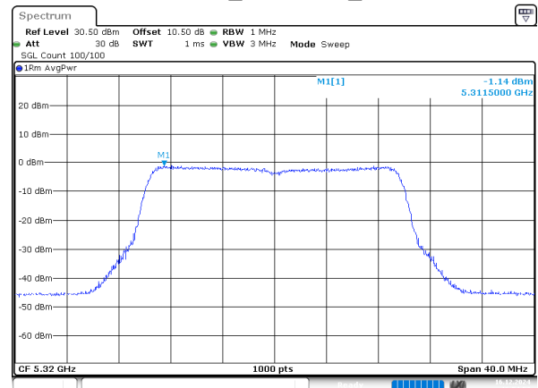
802.11be20_5320MHz_Chain 3
