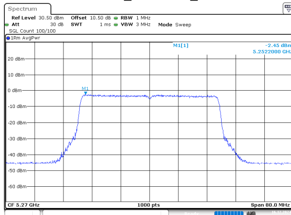
802.11be40_5270MHz_Chain 0
