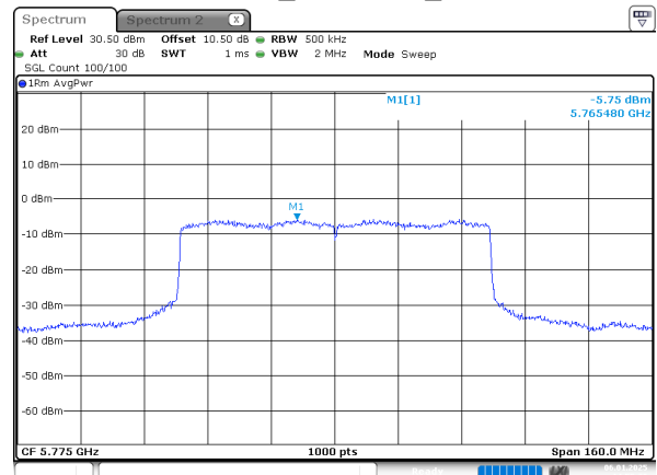
802.11be80_5775MHz_Chain 1
