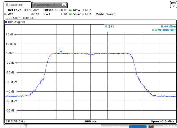
802.11be20_5580MHz_Chain 0
