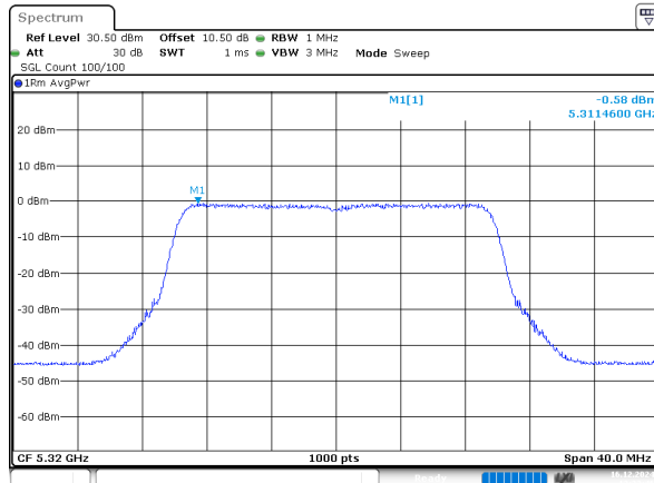
802.11be20_5320MHz_Chain 0
