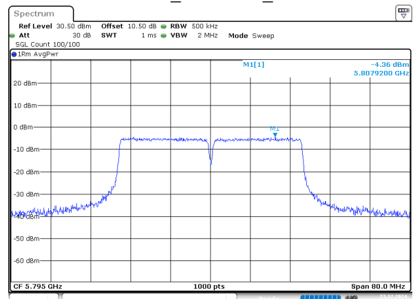
802.11n40_5795MHz_Chain 2
