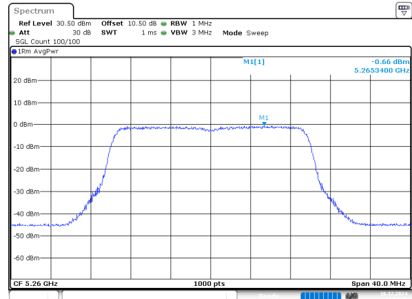
802.11be20_5260MHz_Chain 1
