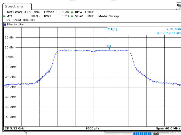
802.11a_5320MHz_Chain 2
