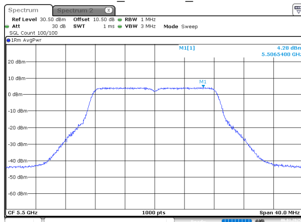
802.11a_5500MHz_Chain 2
