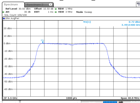
802.11be20_5500MHz_Chain 1
