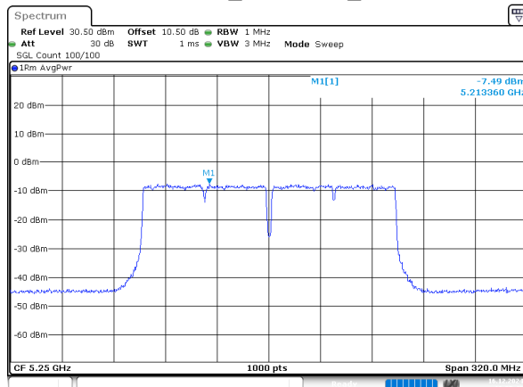
802.11ac160_5250MHz_Chain 2
