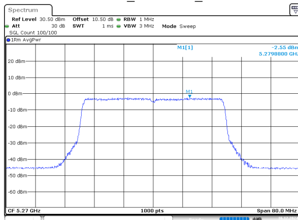
802.11be40_5270MHz_Chain 3
