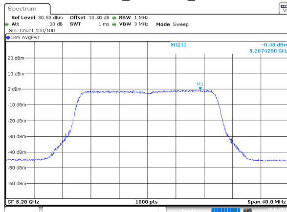
802.11be20_5280MHz_Chain 1
