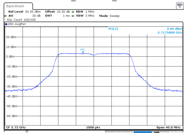
802.11a_5720MHz_Chain 3
