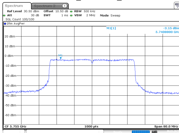
802.11be40_5755MHz_Chain 0
