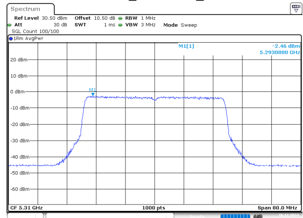
802.11be40_5310MHz_Chain 0
