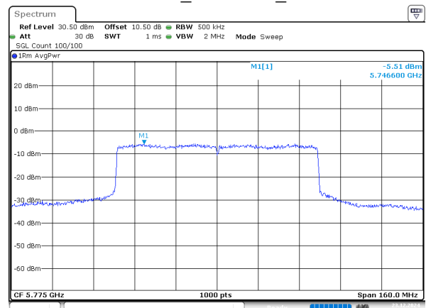
802.11be80_5775MHz_Chain 3
