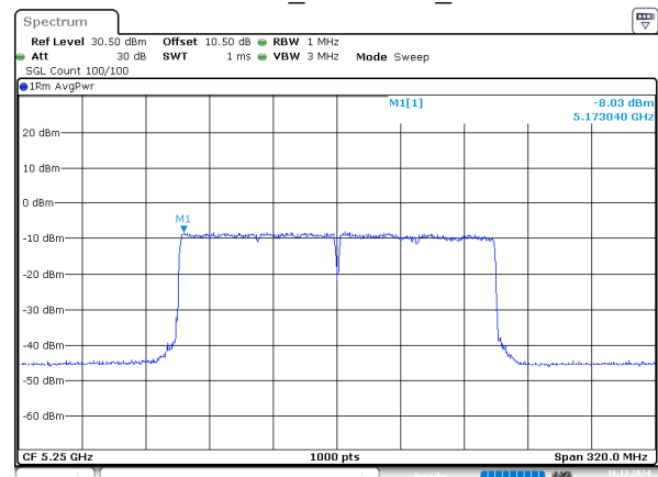
802.11be160_5250MHz_Chain 1
