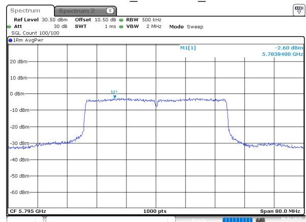
802.11be40_5795MHz_Chain 1
