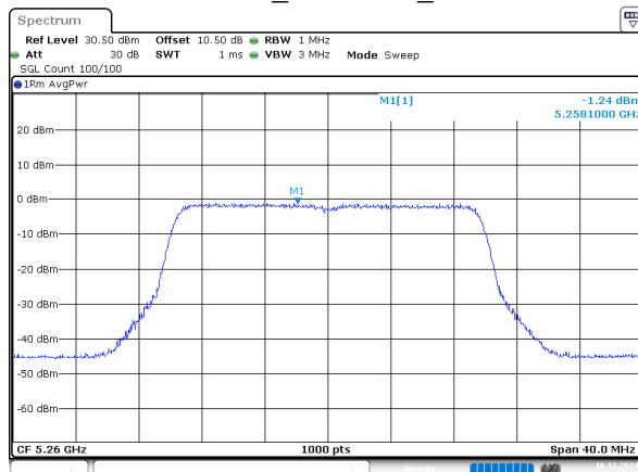
802.11be20_5260MHz_Chain 2
