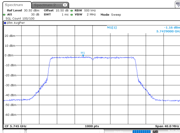
802.11be20_5745MHz_Chain 0
