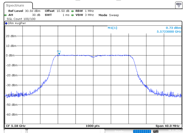
802.11n20_5580MHz_Chain 2
