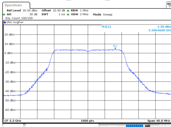
802.11a_5500MHz_Chain 3
