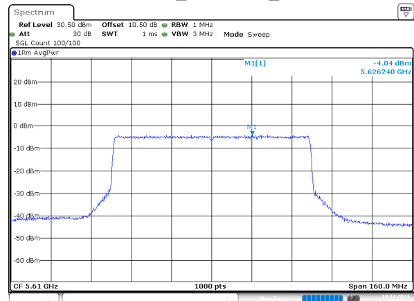
802.11be80_5610MHz_Chain 2
