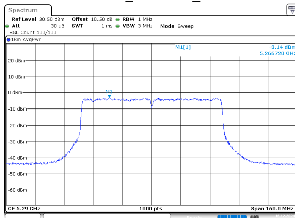
802.11ac80_5290MHz_Chain 2
