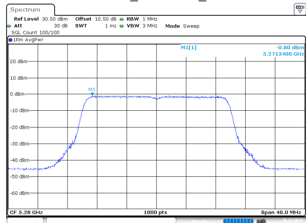
802.11be20_5280MHz_Chain 2
