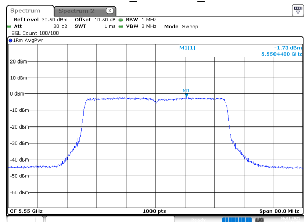
802.11be40_5550MHz_Chain 1
