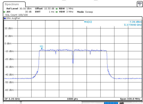
802.11ac160_5250MHz_Chain 3
