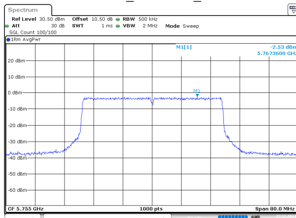
802.11be40_5755MHz_Chain 2
