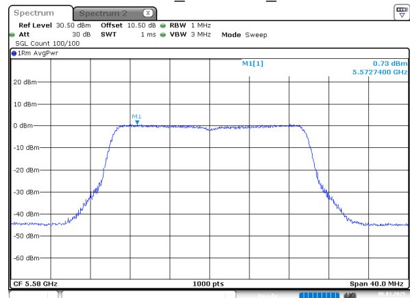
802.11be20_5580MHz_Chain 1
