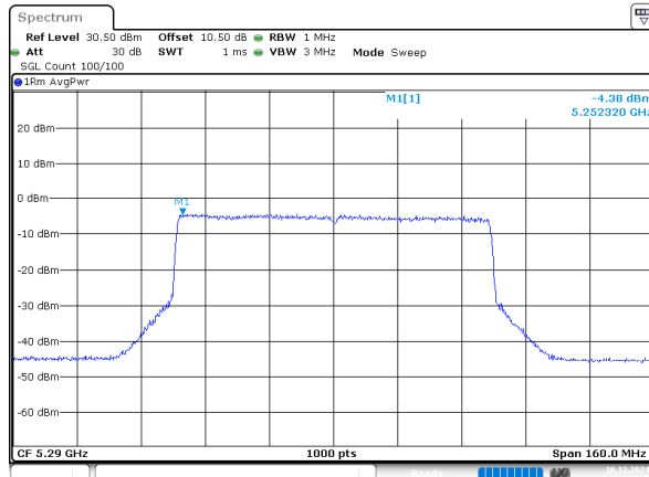
802.11be80_5290MHz_Chain 0
