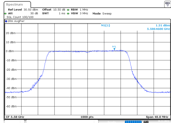
802.11be20_5580MHz_Chain 3
