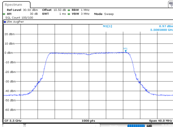
802.11be20_5500MHz_Chain 3
