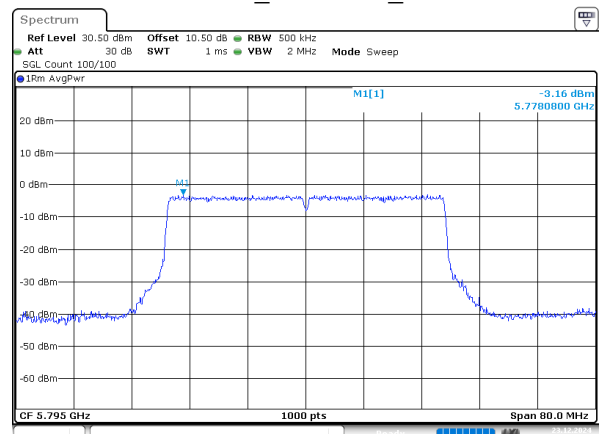
802.11be40_5795MHz_Chain 2
