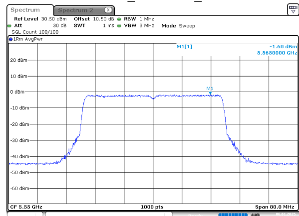
802.11be40_5550MHz_Chain 0
