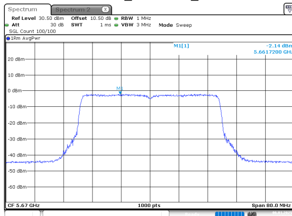
802.11be40_5670MHz_Chain 0
