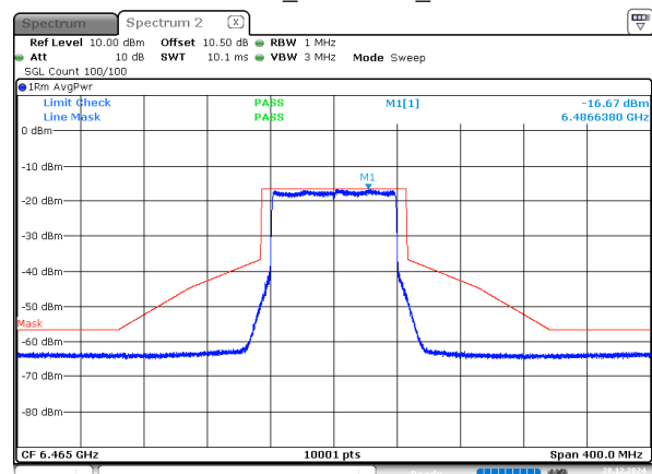
802.11be80 6465MHz Chain 0
