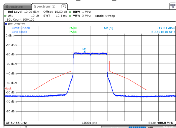
802.11be80 6465MHz Chain 1
