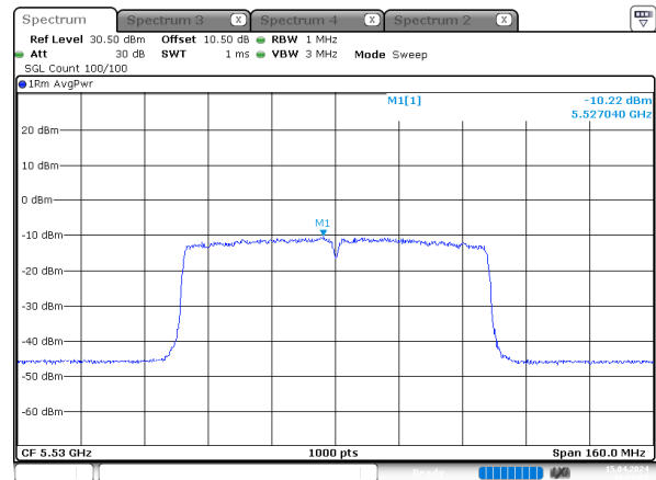
ac80_5530MHz_Chain 1
