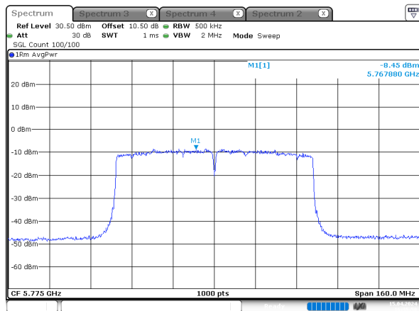
ac80_5775MHz_Chain 2
