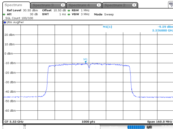
ac80_5530MHz_Chain 2
