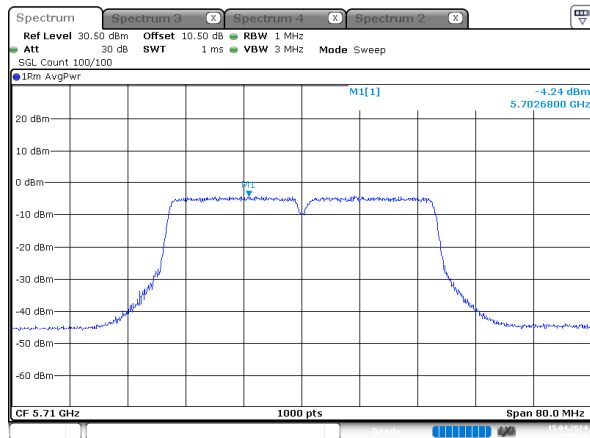
n40_5710MHz_Chain 2
