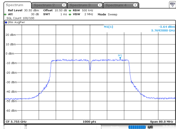
n40_5755MHz_Chain 3
