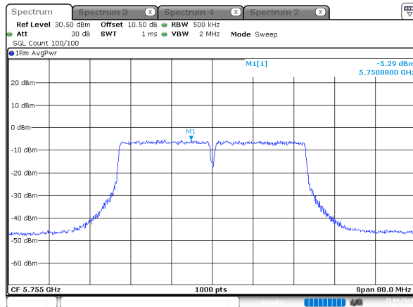
n40_5755MHz_Chain 2
