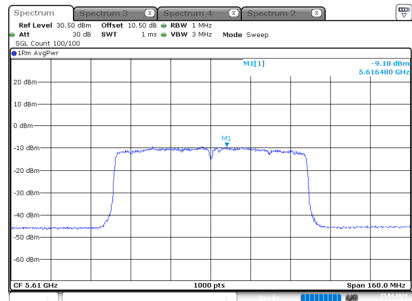
ac80_5610MHz_Chain 1
