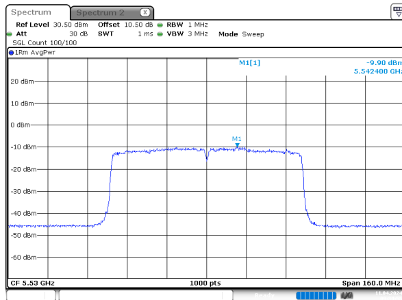
ac80_5530MHz_Chain 0
