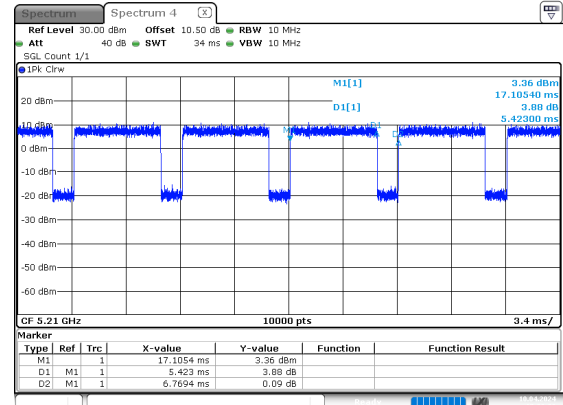
ac80_5210MHz_Chain 0
