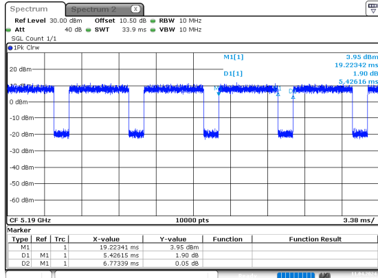
n40_5190MHz_Chain 0
