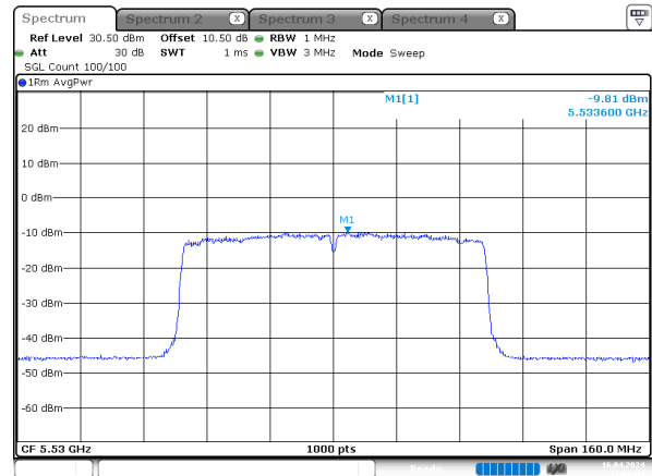
ac80_5530MHz_Chain 3
