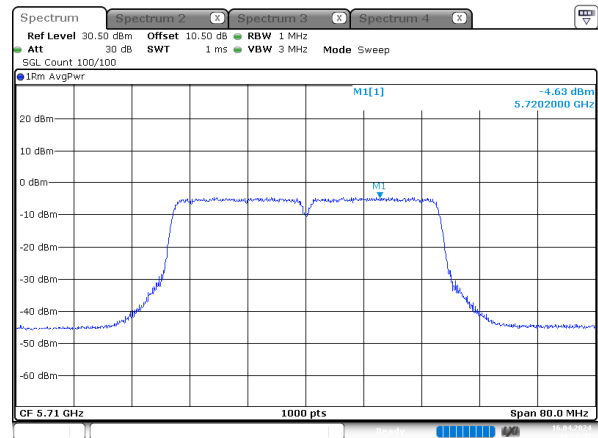
n40_5710MHz_Chain 3
