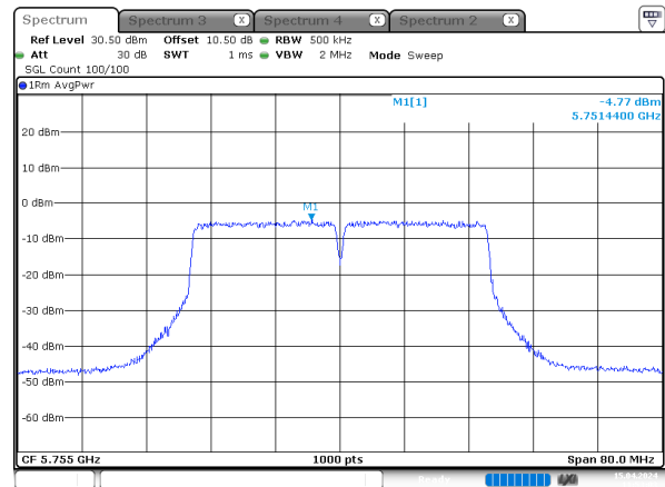
n40_5755MHz_Chain 1
