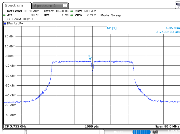
n40_5755MHz_Chain 0
