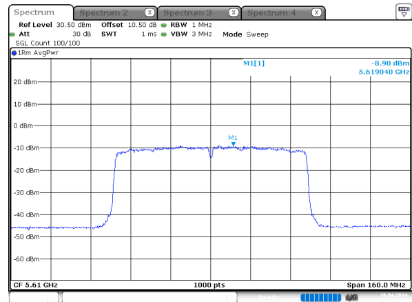
ac80_5610MHz_Chain 3
