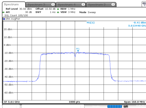
ac80_5610MHz_Chain 2
