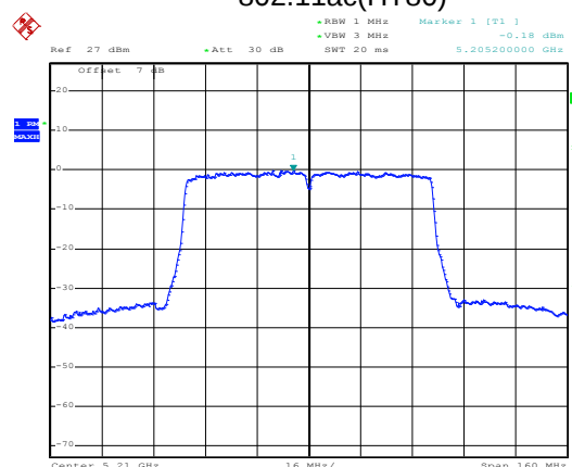
802.11ac(HT80)
