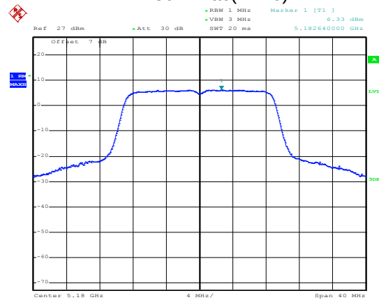
802.11ac(HT20)
