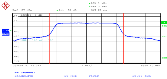
802.11a
