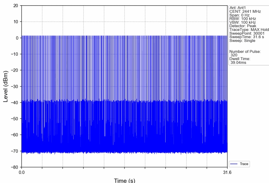
Pi/4DQPSK_2DH5_HOPP_Ant1_NTNV
