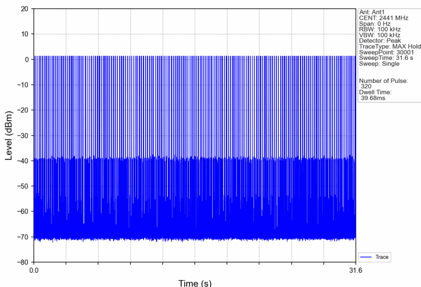
Pi/4DQPSK_2DH3_HOPP_Ant1_NTNV
