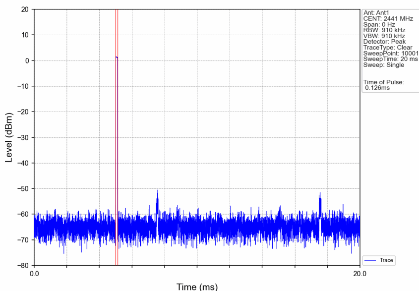
GFSK_DH5_HOPP_Ant1_NTNV
