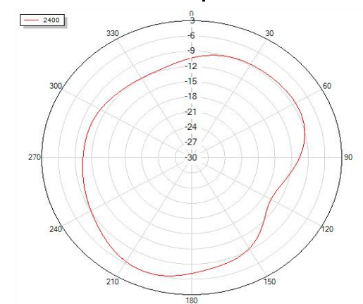
Theta=90 freq=2400MHz
