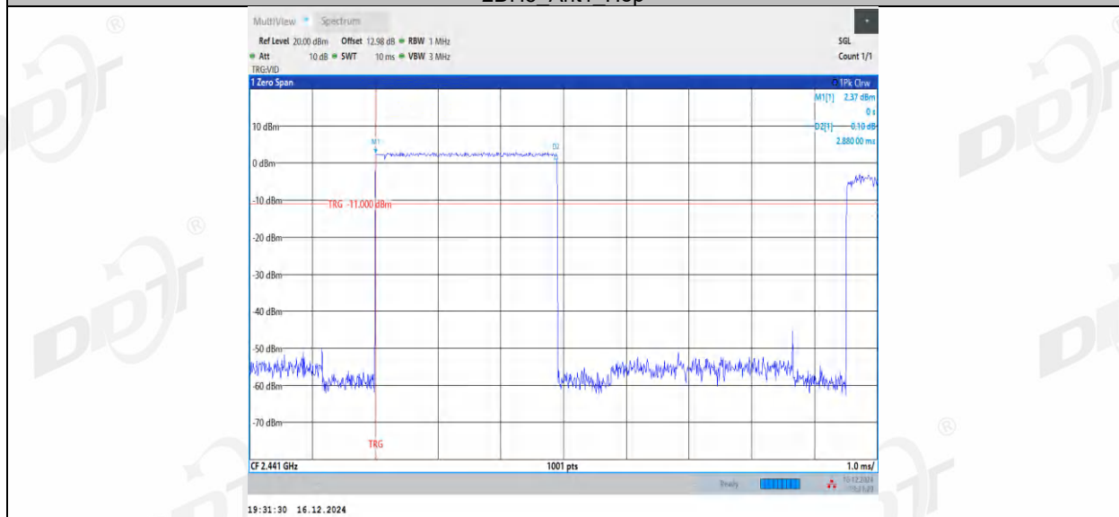
2DH5_Ant1_Hop
