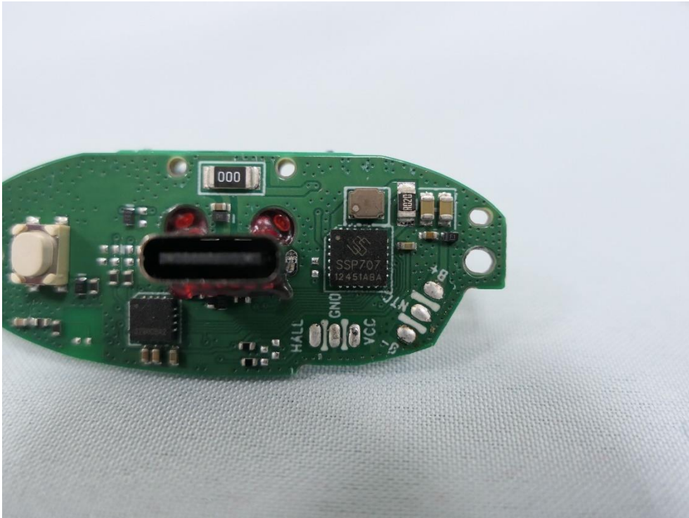
(31) EUT Photo
