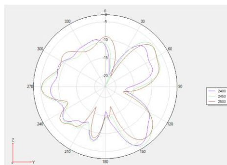
Phi 90 2D 图
