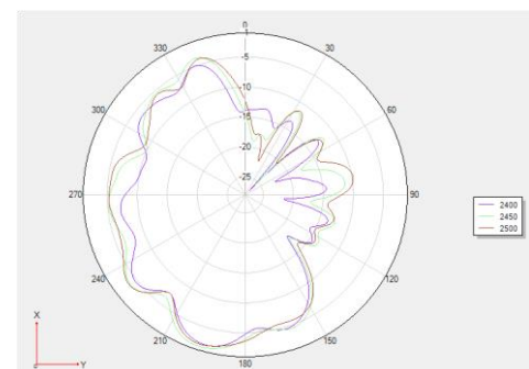
Theta 90 2D 图
