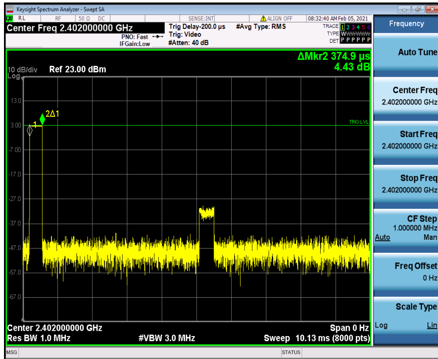
DH1_Ant1_Hop_2402
