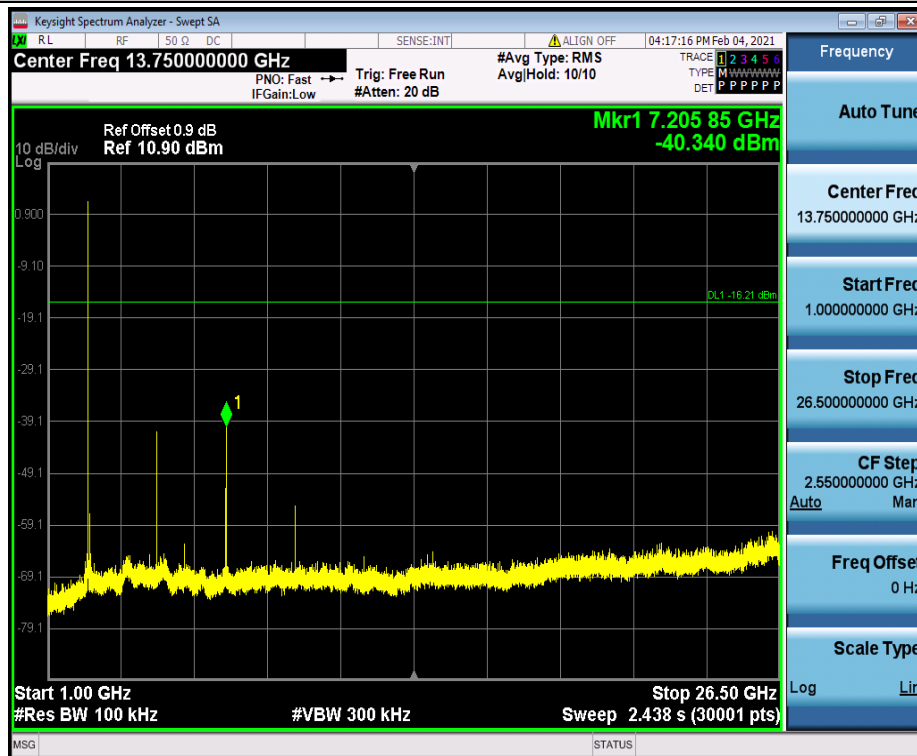
2DH5_Ant1_2402_1000~26500
