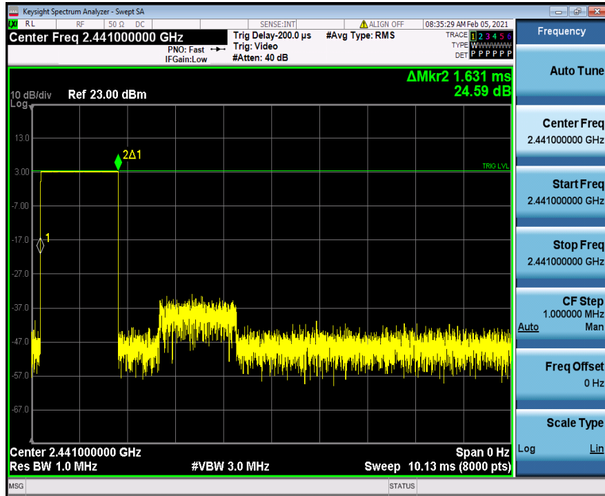
DH3_Ant1_Hop_2441
