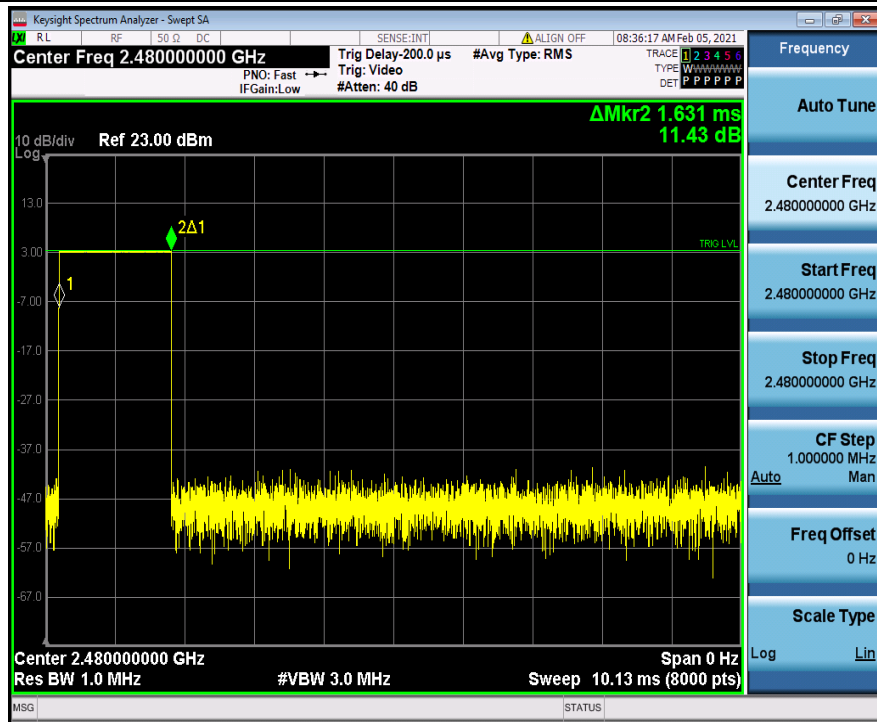
DH3_Ant1_Hop_2480
