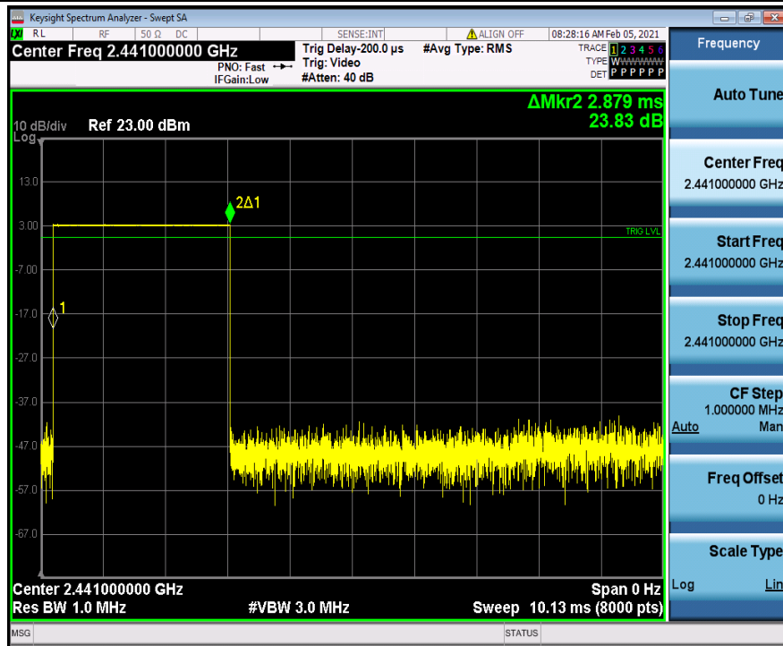
DH5_Ant1_Hop_2441
