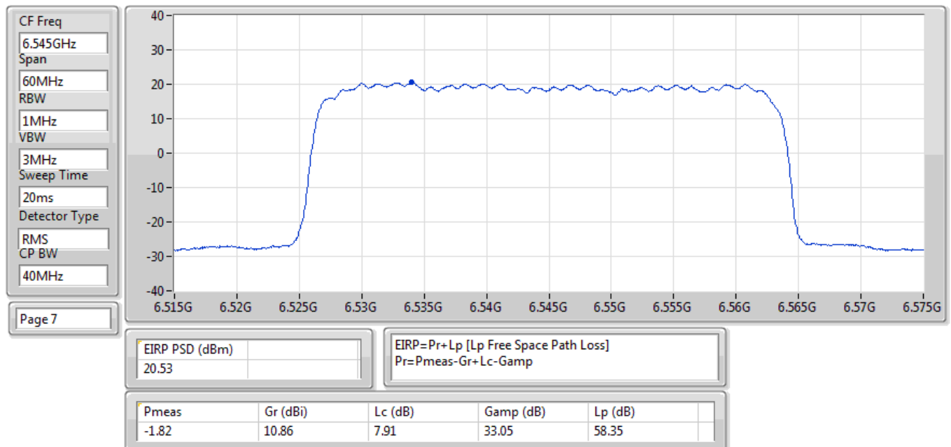
EIRP PSD;Band:6.7G;QPSK40;BWch:40MHz;Nss:1;Nant:2;Ch:6545MHz;TX
