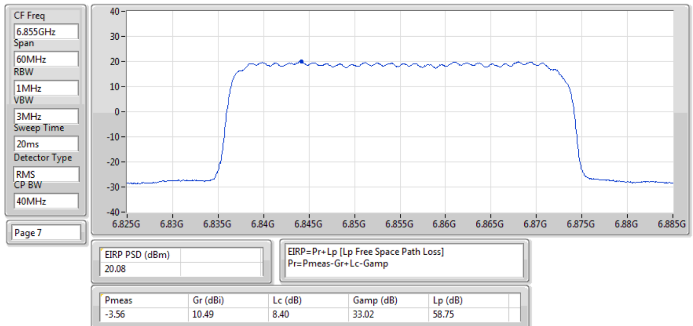
EIRP PSD;Band:6.7G;QPSK40;BWch:40MHz;Nss:1;Nant:2;Ch:6855MHz;TX
