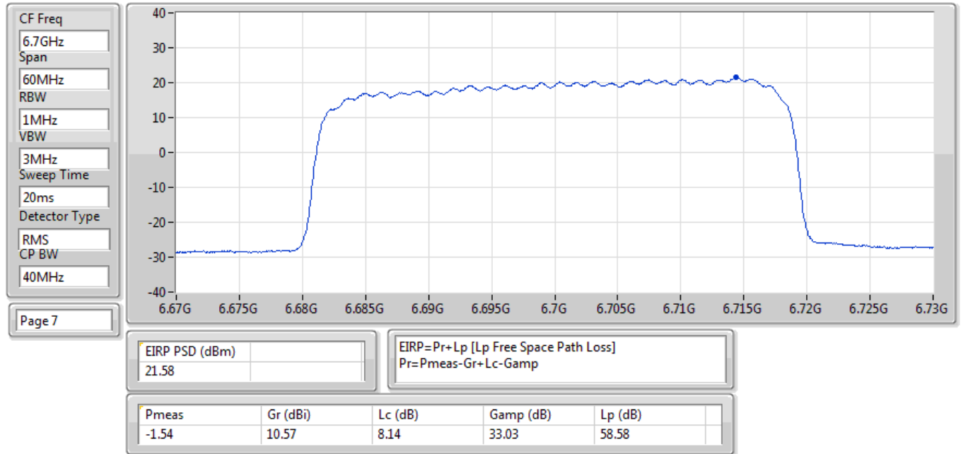
EIRP PSD;Band:6.7G;QPSK40;BWch:40MHz;Nss:1;Nant:2;Ch:6700MHz;TX
