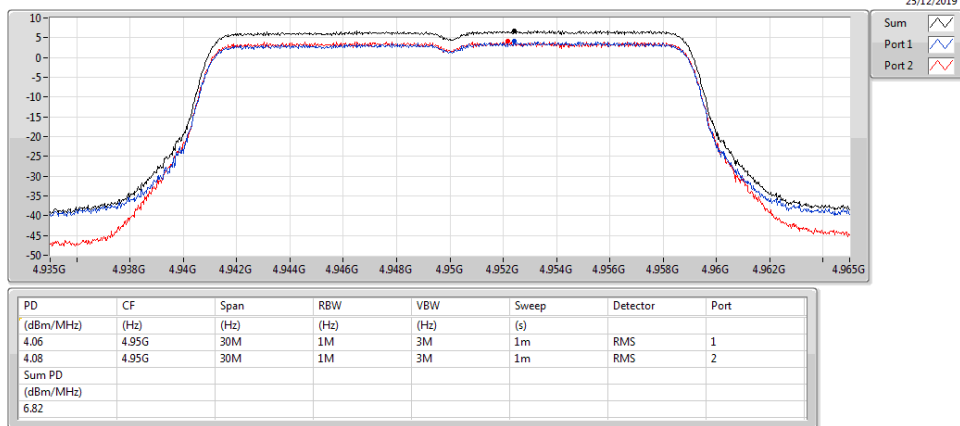
4.94-4.99GHz_802.11j_20MHz_Nss1_2TX 4950MHz
