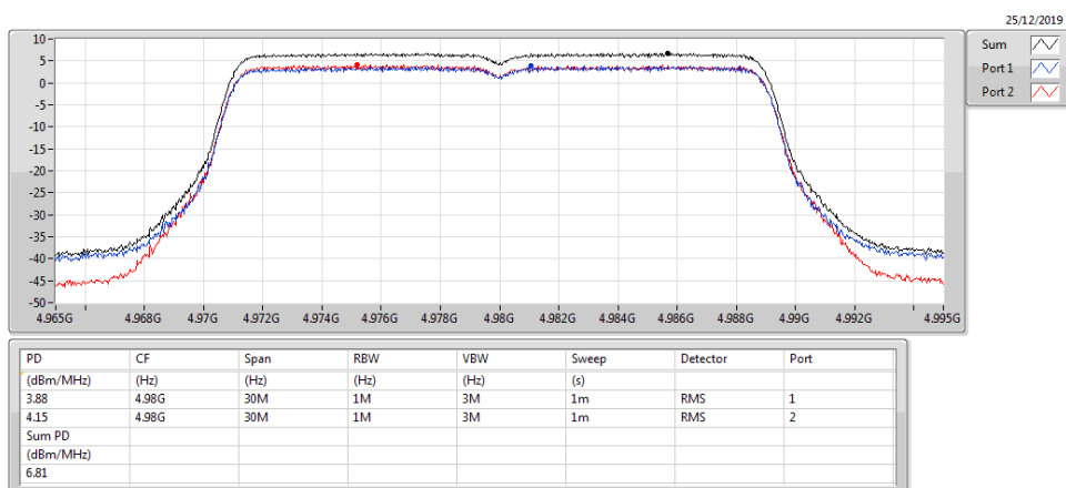
4.94-4.99GHz_802.11j_20MHz_Nss1_2TX 4980MHz
