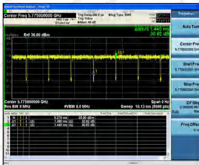
11AC80SISO_Ant1_5775
