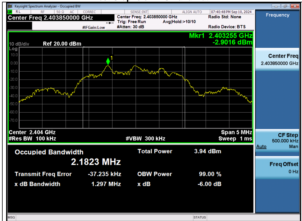
Test_Graph_2.4G_ANT1_2403.85_DTSBW
