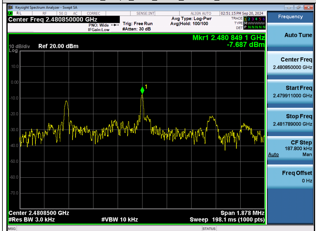
Test_Graph_2.4G_ANT1_2480.85_PSD
