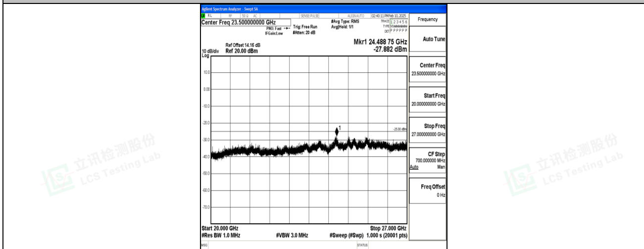
Band7_20MHz_QPSK_20850_1RB#0_20000~27000_20000~27000
