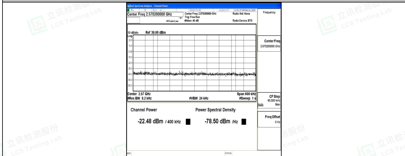
Band7_20MHz_QPSK_21350_100RB#0_Final1
