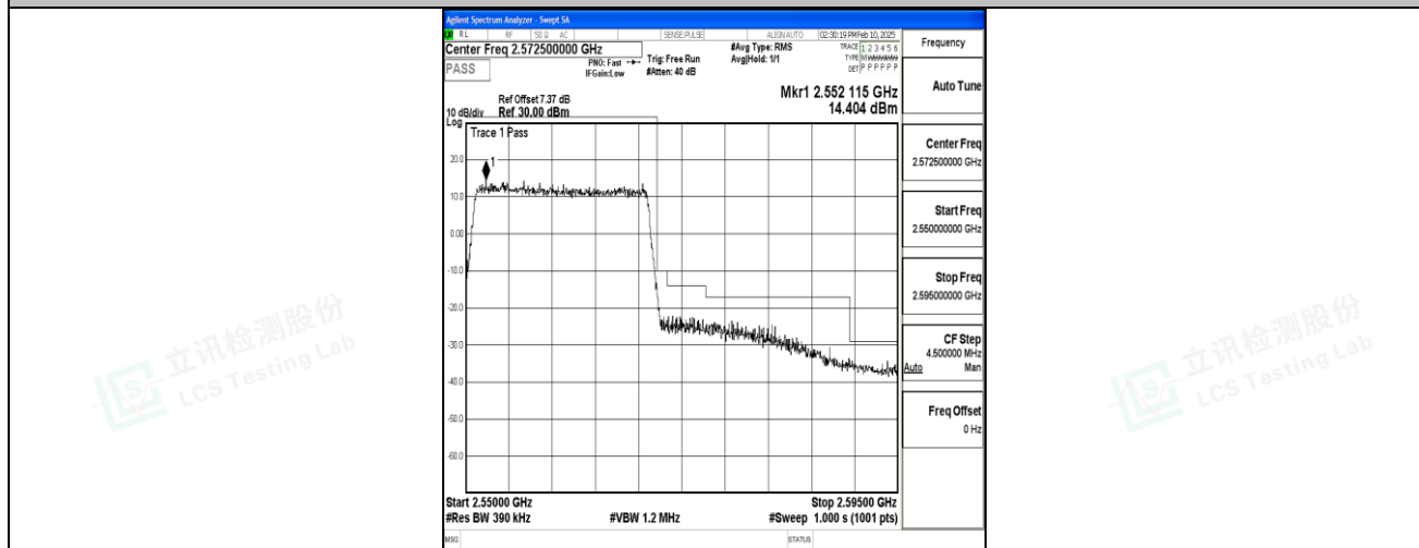
Band7_20MHz_QPSK_21350_100RB#0
