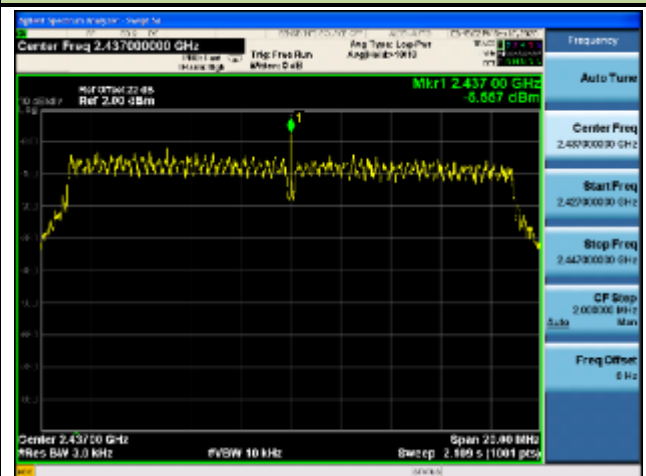
802.11 n-20M CH06 (2437MHz)
