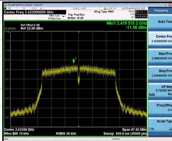
11N40_Ant2_2422
