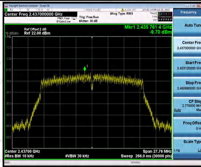
11N20_Ant2_2437
