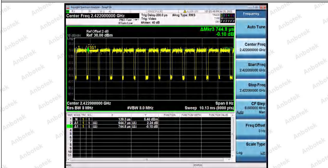
11N40_Ant1_2422
