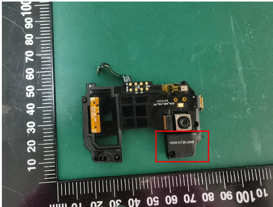
BT/Wi-Fi/GNSS ANT
