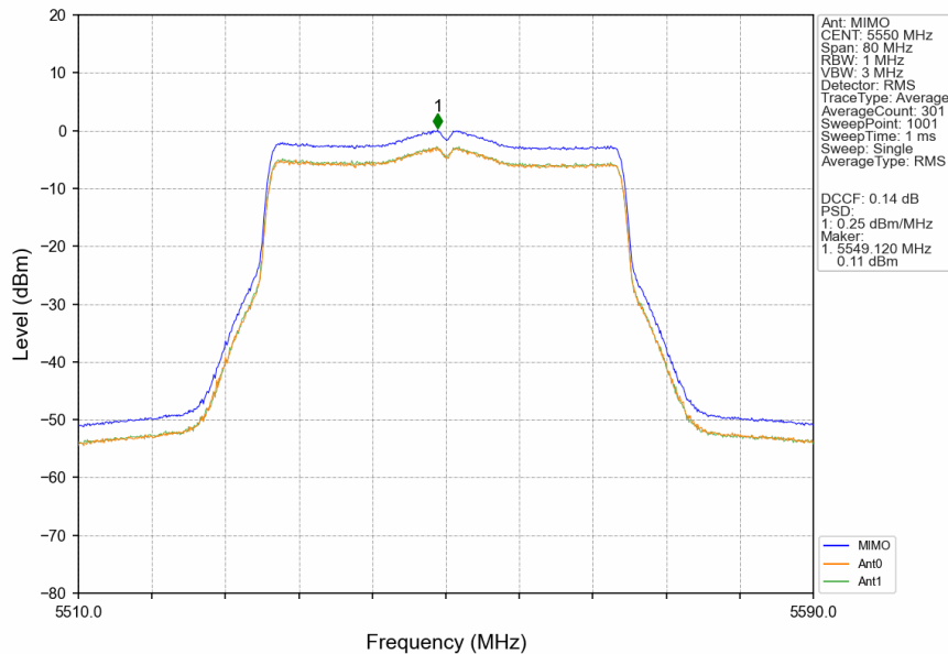
802.11be(EHT40)_MCH_5550MHz_SU_ / _MIMO_NTNV
