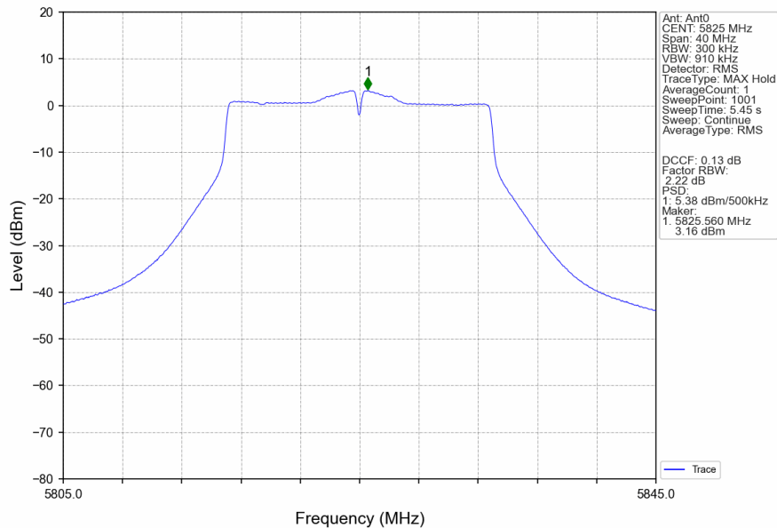
802.11ac(VHT20)_HCH_5825MHz_Ant0_NTNV
