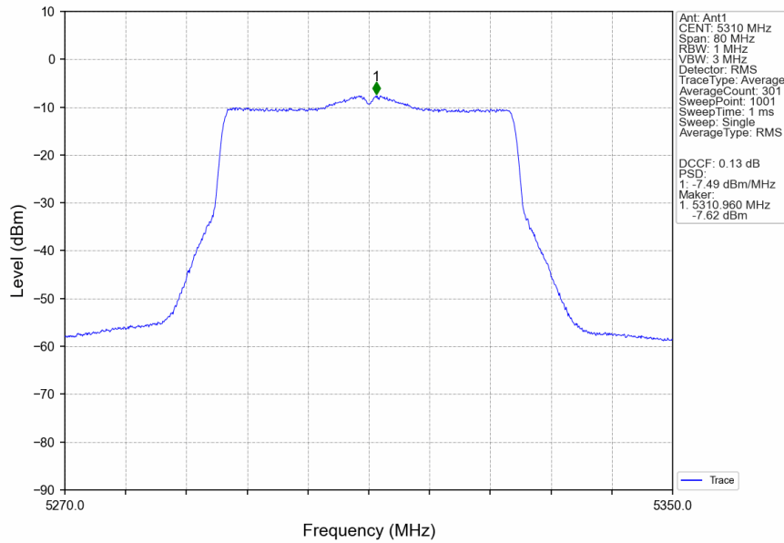
802.11be(EHT40)_HCH_5310MHz_SU_ / _MIMO_NTNV
