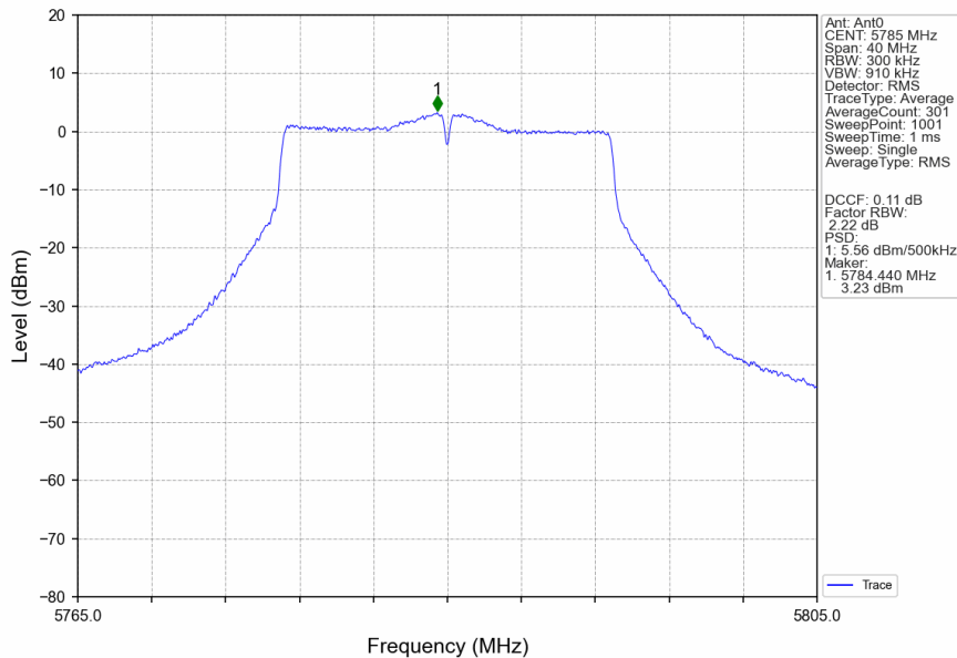
802.11n(HT20)_MCH_5785MHz_Ant0_NTNV
