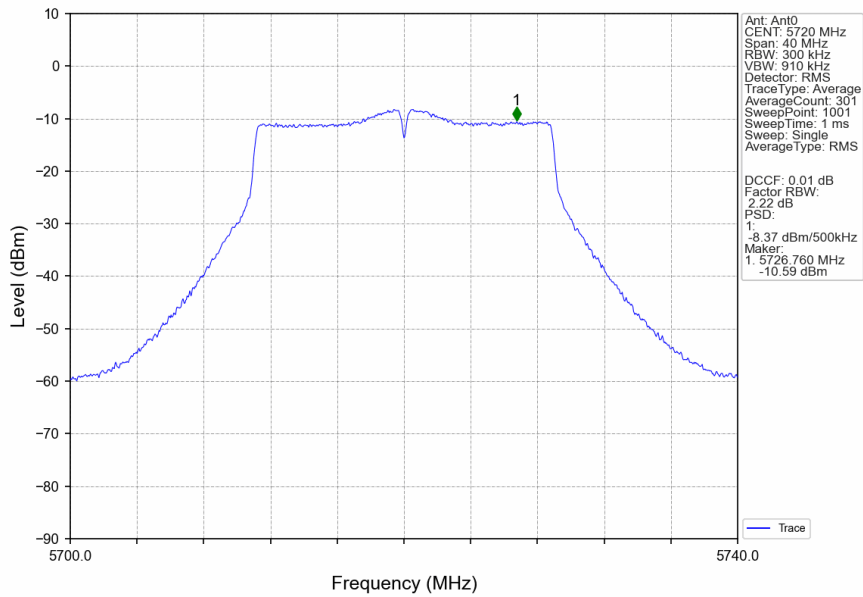
802.11n(HT20)_HCH_5720MHz_Ant0_NTNV
