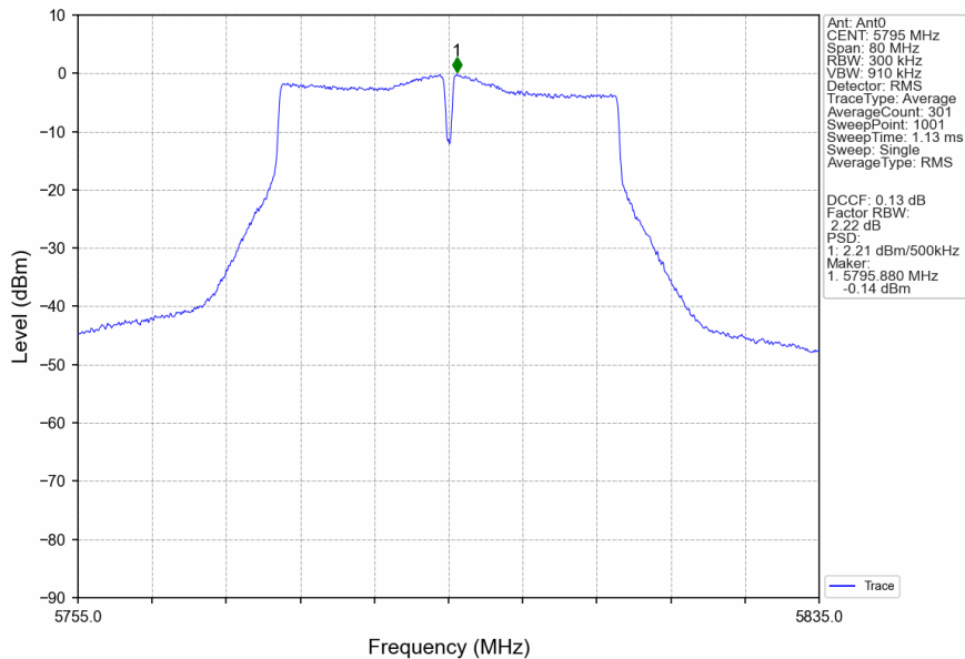
802.11n(HT40)_HCH_5795MHz_Ant0_NTNV
