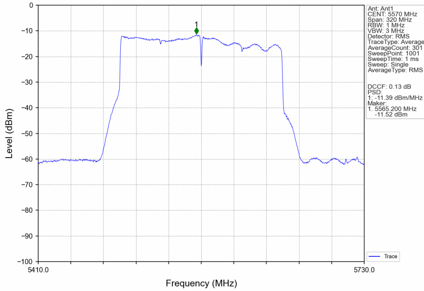
802.11be(EHT160)_MCH_5570MHz_SU_ / _MIMO_NTNV
