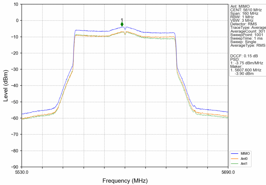
802.11be(EHT80)_HCH_5610MHz_SU_ / _MIMO_NTNV
