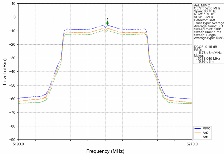
802.11be(EHT40)_HCH_5230MHz_SU_ / _MIMO_NTNV
