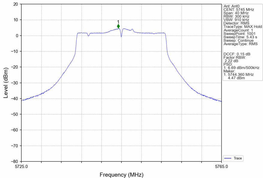
802.11ac(VHT20)_LCH_5745MHz_Ant0_NTNV
