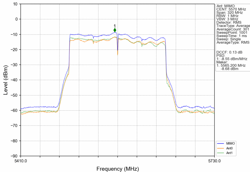
802.11be(EHT160)_MCH_5570MHz_SU_ / _MIMO_NTNV
