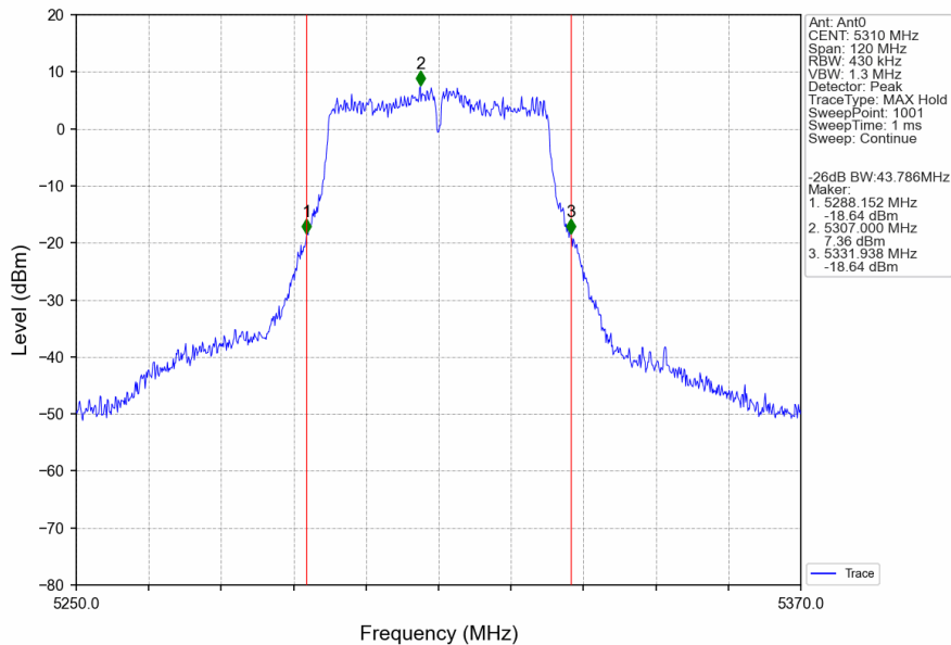
802.11ac(VHT40)_HCH_5310MHz_Ant0_NTNV
