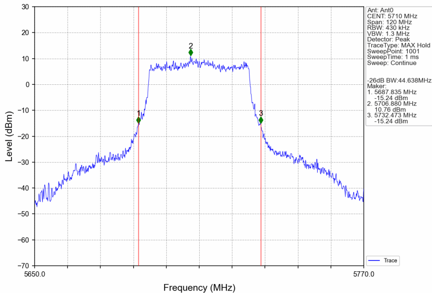
802.11ac(VHT40)_HCH_5710MHz_Ant0_NTNV
