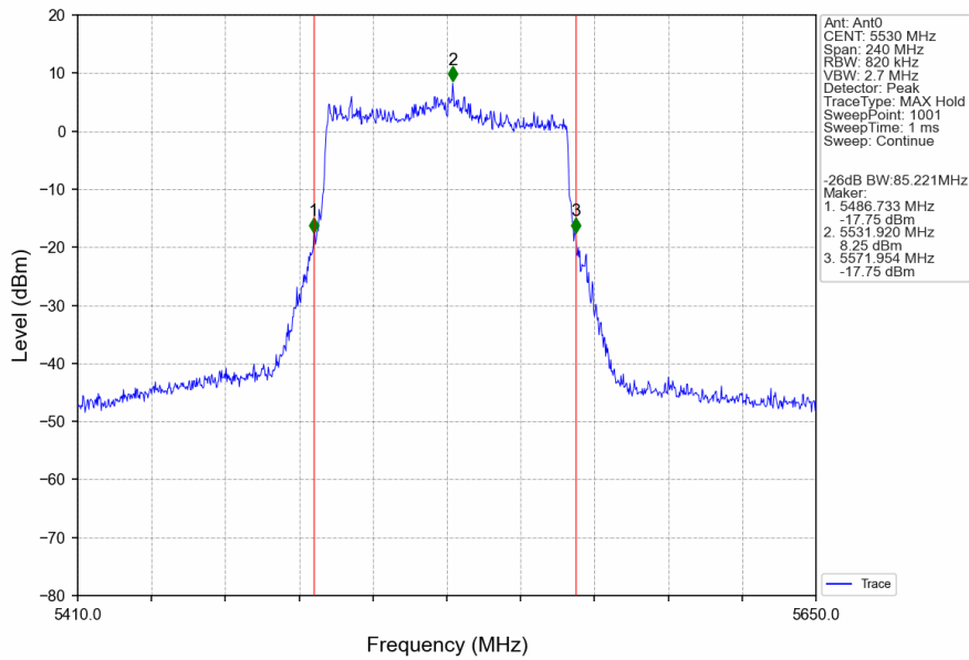
802.11ax(HEW80)_LCH_5530MHz_SU_ / _Ant0_NTNV
