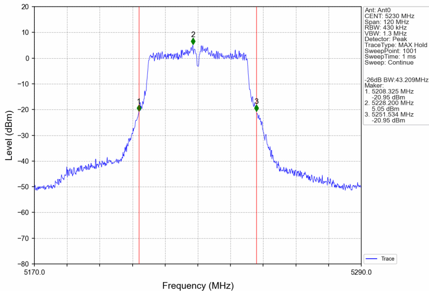
802.11ac(VHT40)_HCH_5230MHz_Ant0_NTNV
