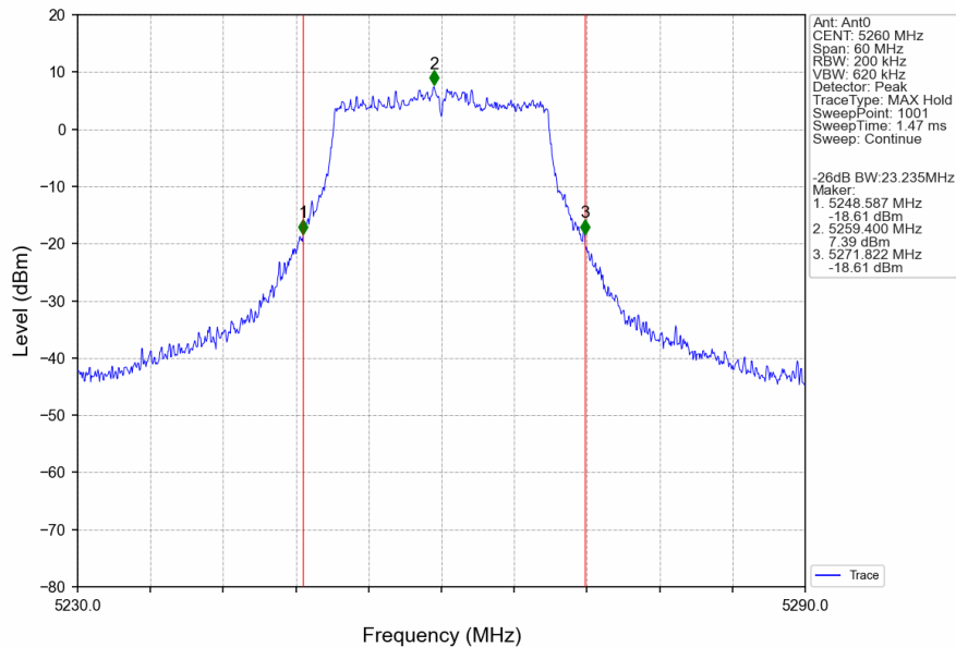
802.11ac(VHT20)_LCH_5260MHz_Ant0_NTNV
