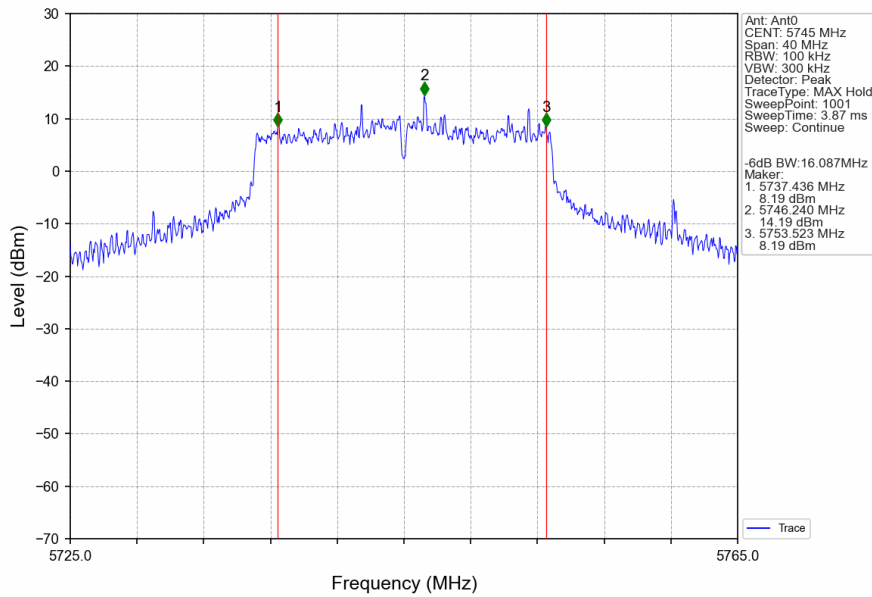
802.11n(HT20)_LCH_5745MHz_Ant0_NTNV
