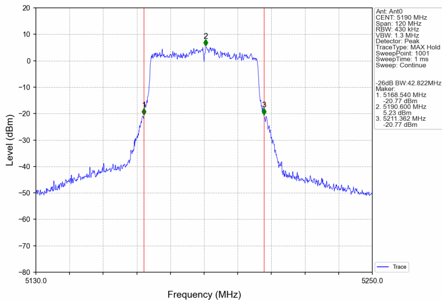
802.11ax(HEW40)_LCH_5190MHz_SU_ / _Ant0_NTNV
