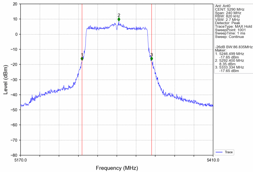
802.11ac(VHT80)_MCH_5290MHz_Ant0_NTNV
