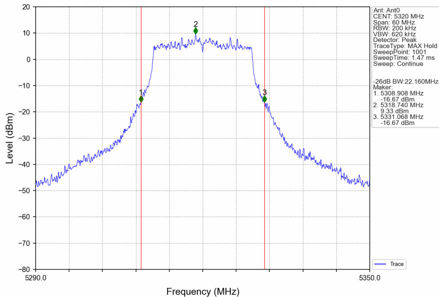
802.11ac(VHT20)_HCH_5320MHz_Ant0_NTNV
