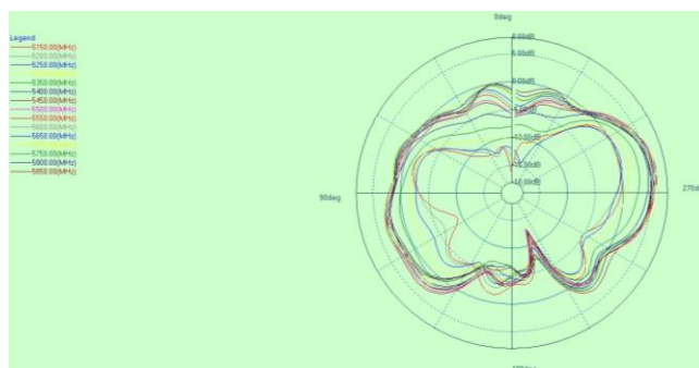
theta=90deg
