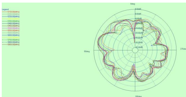
phi=0deg
