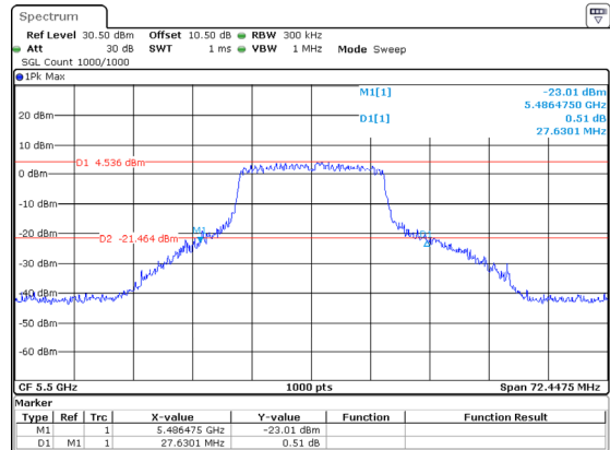
802.11ac20_5500MHz_Chain 1 27.630MHz
