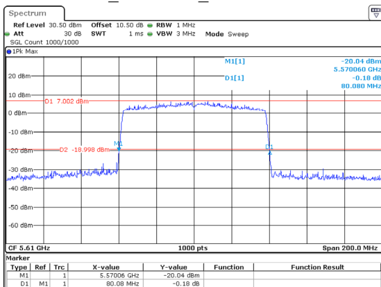
802.11ac80_5610MHz_Chain 2 80.080MHz
