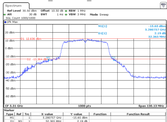
802.11ac40_5310MHz_Chain 2 52.365MHz
