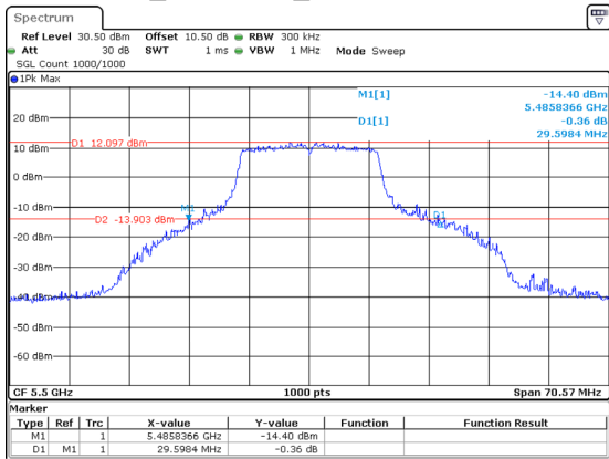
802.11a_5500MHz_Chain 0 29.598MHz
