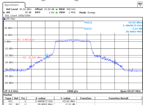
802.11ac20_5500MHz_Chain 2 28.900MHz
