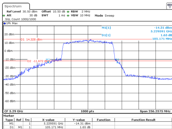
802.11ac80_5290MHz_Chain 2 105.171MHz
