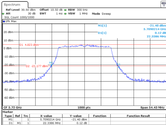
802.11ac20_5720MHz_Chain 0 22.339MHz
