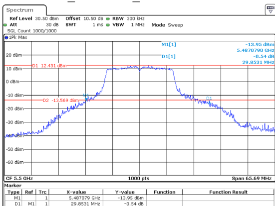
802.11a_5500MHz_Chain 1 29.853MHz
