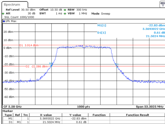
802.11ac20_5580MHz_Chain 2 21.502MHz
