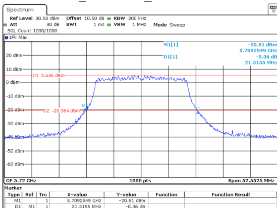
802.11ac20_5720MHz_Chain 1 21.515MHz
