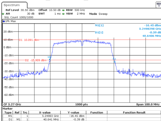
802.11ac40_5270MHz_Chain 1 40.641MHz
