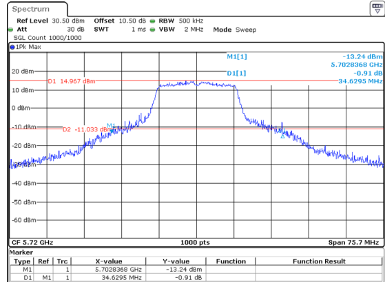
802.11a_5720MHz_Chain 1 34.630MHz
