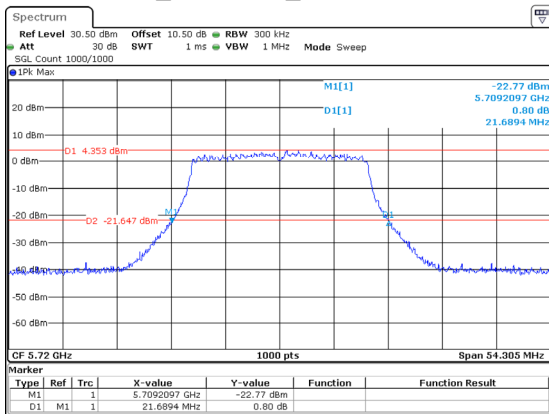
802.11ac20_5720MHz_Chain 2 21.689MHz
