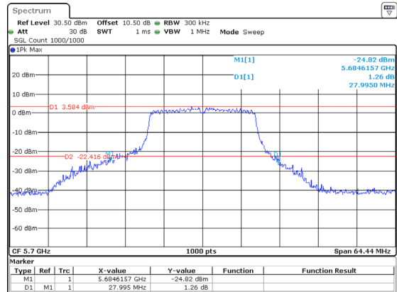
802.11ac20_5700MHz_Chain 2 27.995MHz
