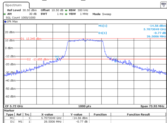
802.11a_5720MHz_Chain 2 26.501MHz
