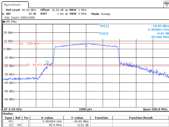
802.11ac80_5530MHz_Chain 1 99.900MHz
