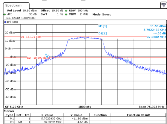
802.11a_5720MHz_Chain 0 37.323MHz
