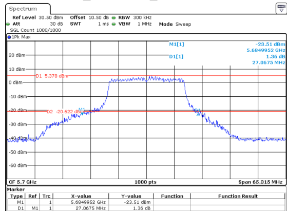
802.11ac20_5700MHz_Chain 1 27.067MHz
