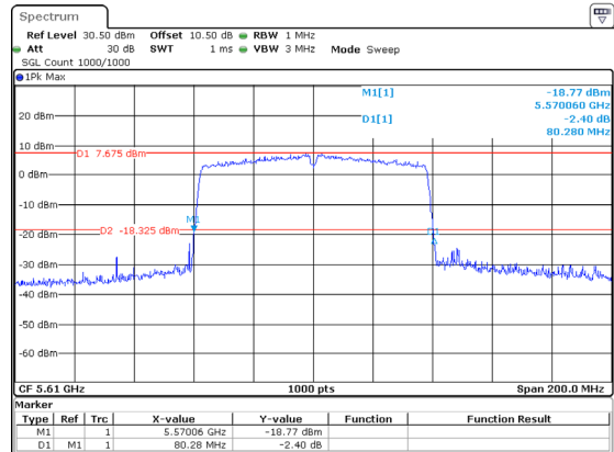
802.11ac80_5610MHz_Chain 1 80.280MHz
