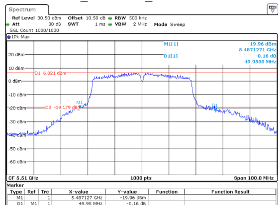
802.11ac40_5510MHz_Chain 2 49.950MHz
