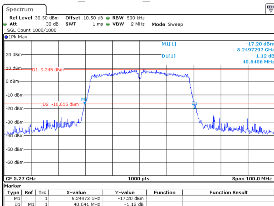
802.11ac40_5270MHz_Chain 2 40.641MHz
