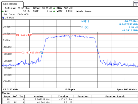
802.11ac40_5270MHz_Chain 0 41.341MHz
