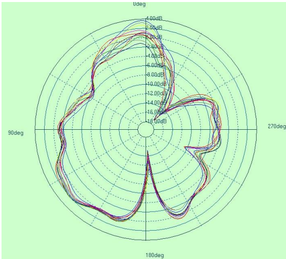
2. 4G phi=0deg
