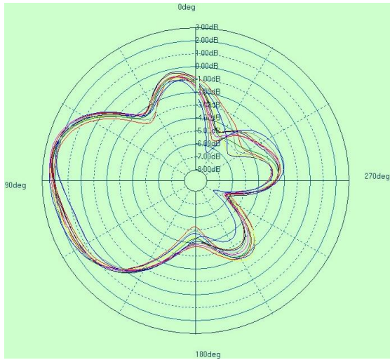
2.4G theta=90deg
