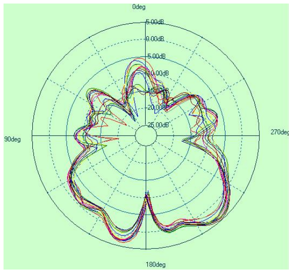
5G phi=0deg
