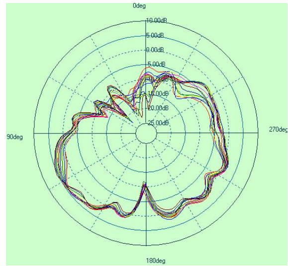
5G phi=90deg
