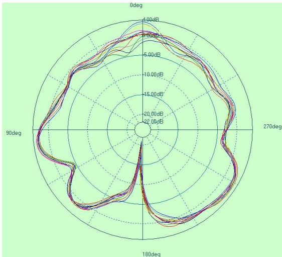
2. 4G phi=90deg
