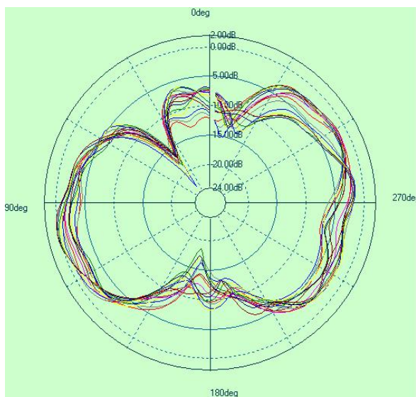
5G theta=90deg
