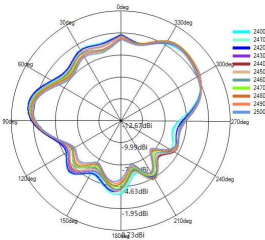
2.4G phi=0deg
