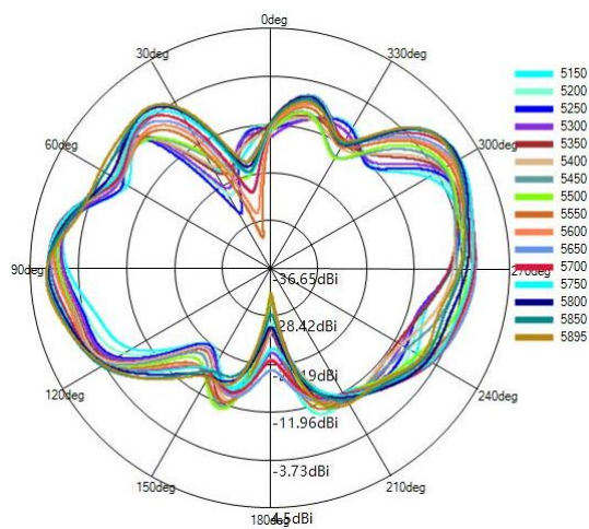
5G phi=90deg
