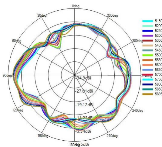
5G phi=0deg
