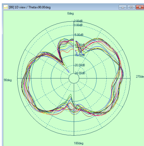
5G theta=90deg
