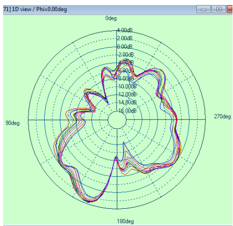
2.4G phi=0deg
