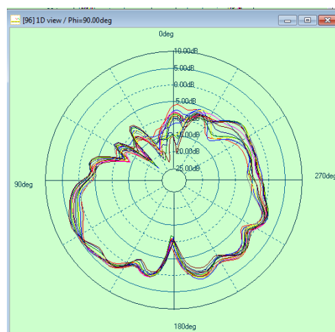
5G phi=90deg
