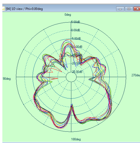
5G phi=0deg
