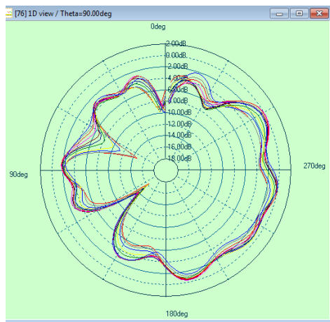
2.4G theta=90deg
