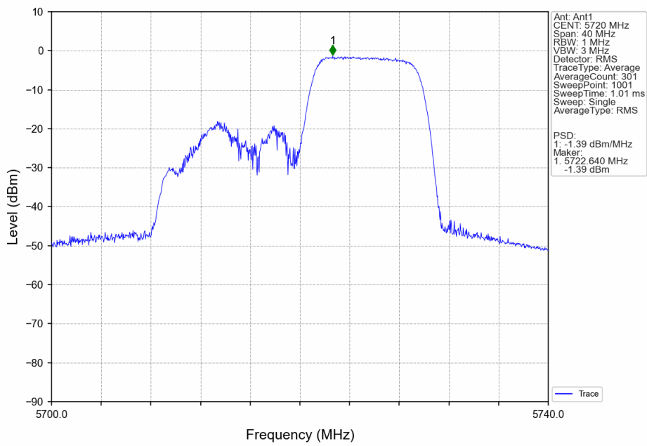
802.11ax(HEW20)_HCH_5720MHz_RU106_Left_Ant1_NTNV
