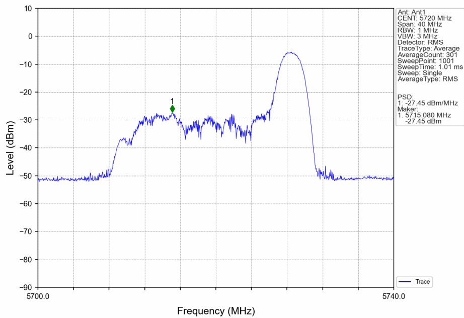
802.11ax(HEW20)_HCH_5720MHz_RU26_Left_Ant1_NTNV
