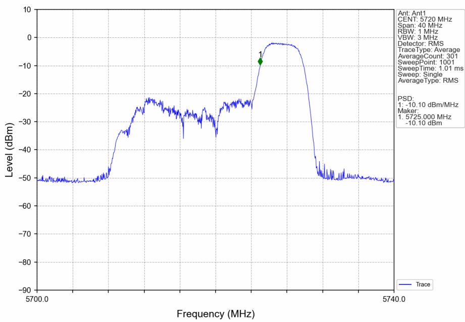
802.11ax(HEW20)_HCH_5720MHz_RU52_Left_Ant1_NTNV
