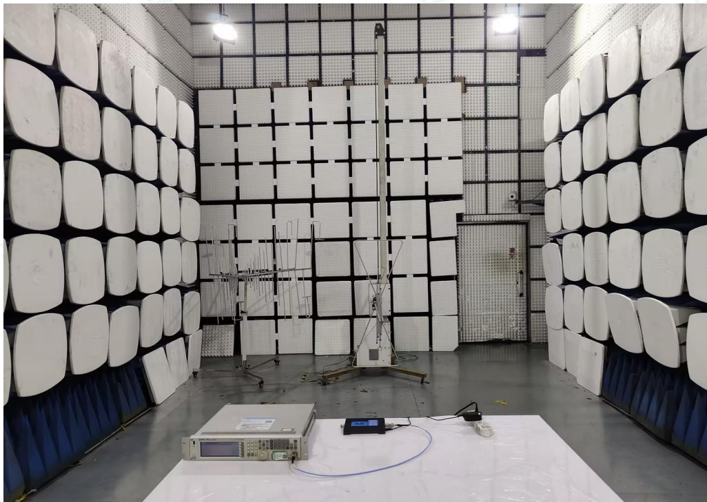
Fig. 1 (Below 1GHz)
