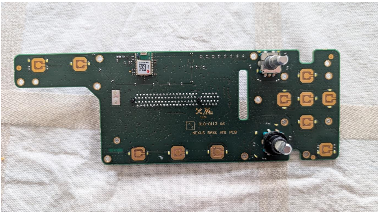
HMI PCA front
