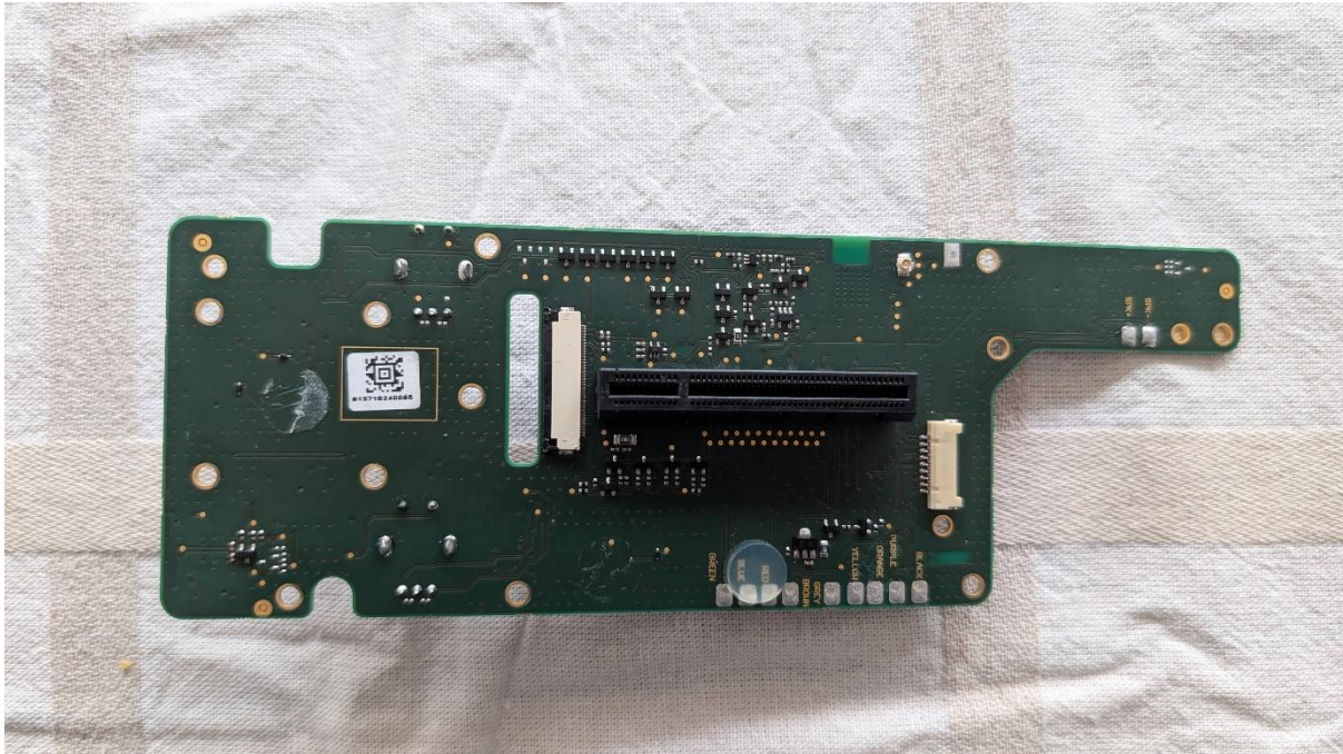
HMI PCA rear
