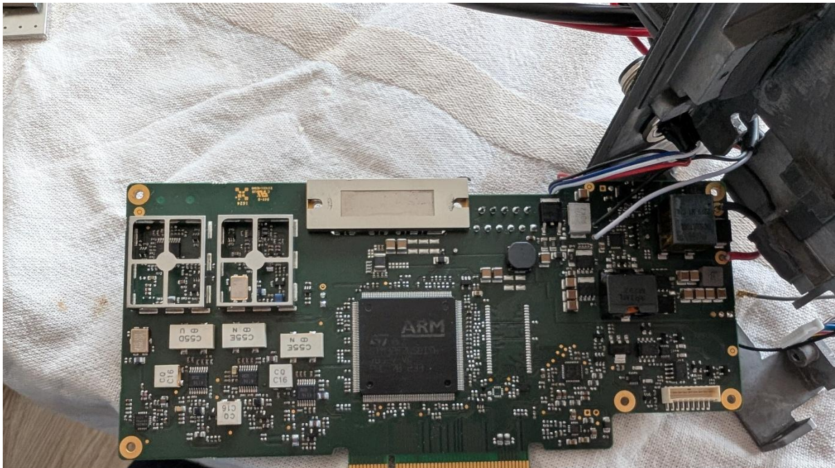
Main PCA bottom without cans
