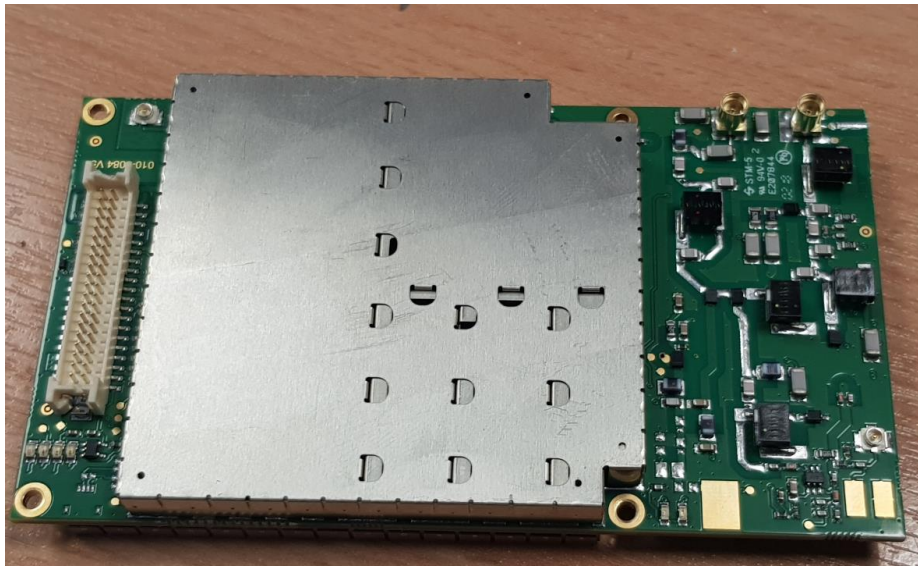
1. PCB Top
