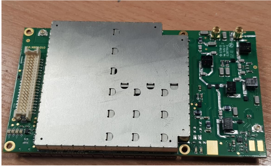
1. PCB Top
