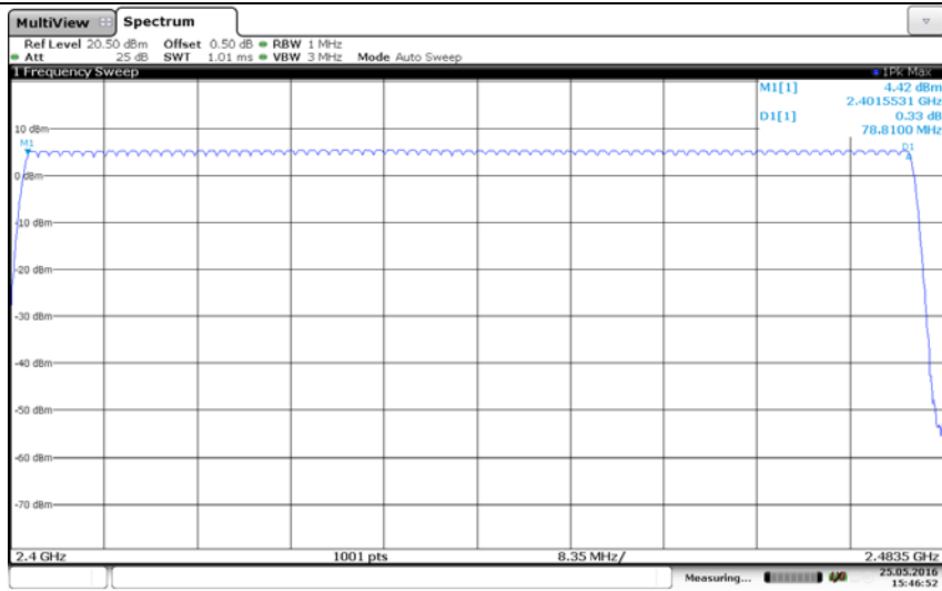
GFSK
