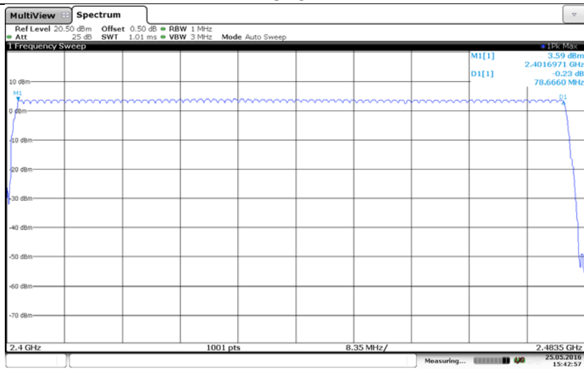
\pi/4 DQPSK
