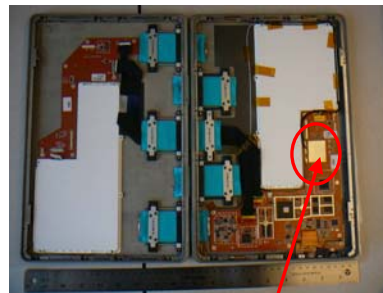
Embedded RF Module
