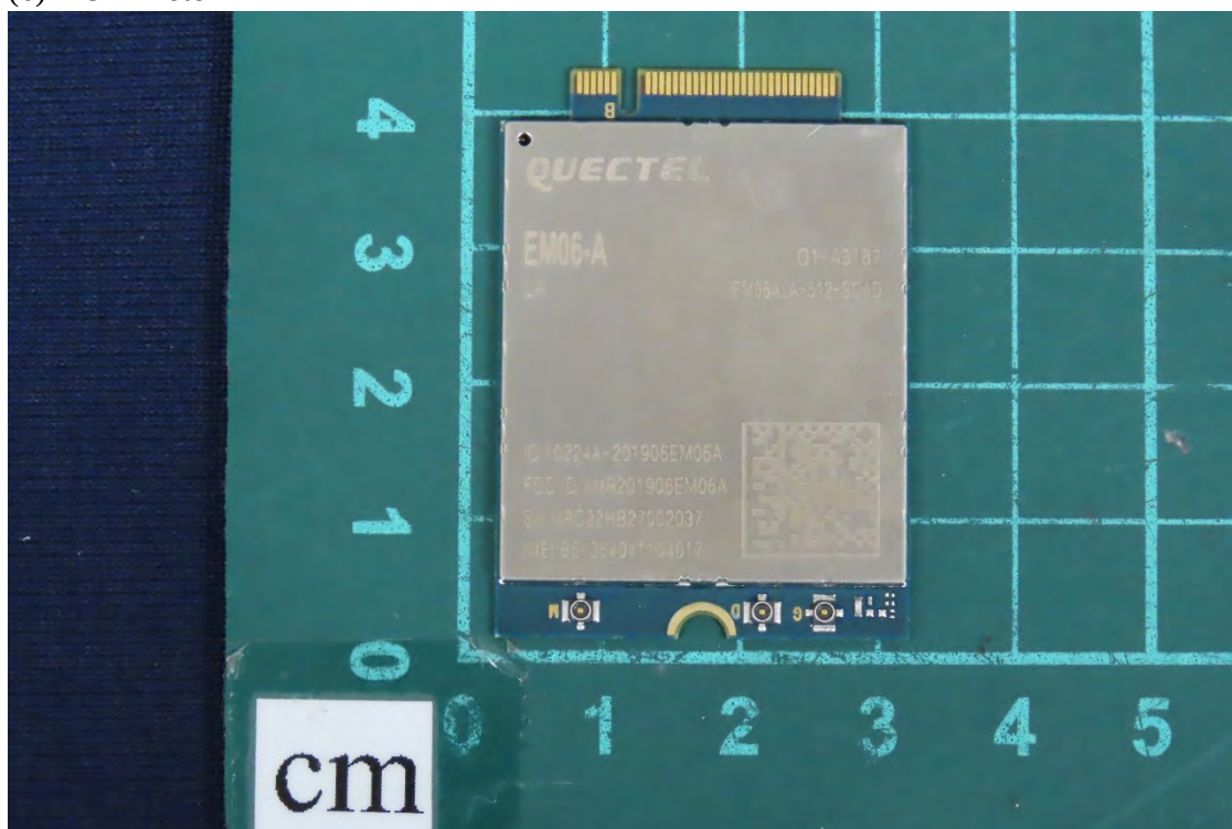
(6) EUT Photo
