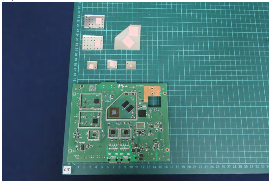
(33) EUT Photo
