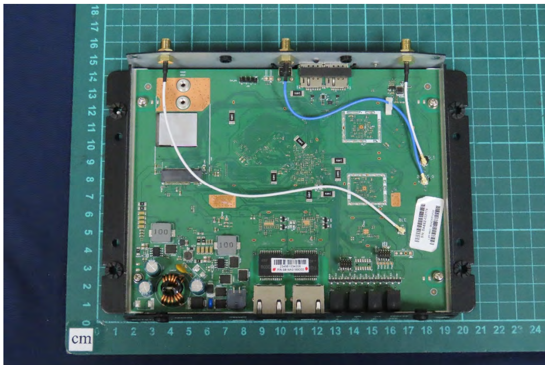
(48) EUT Photo
