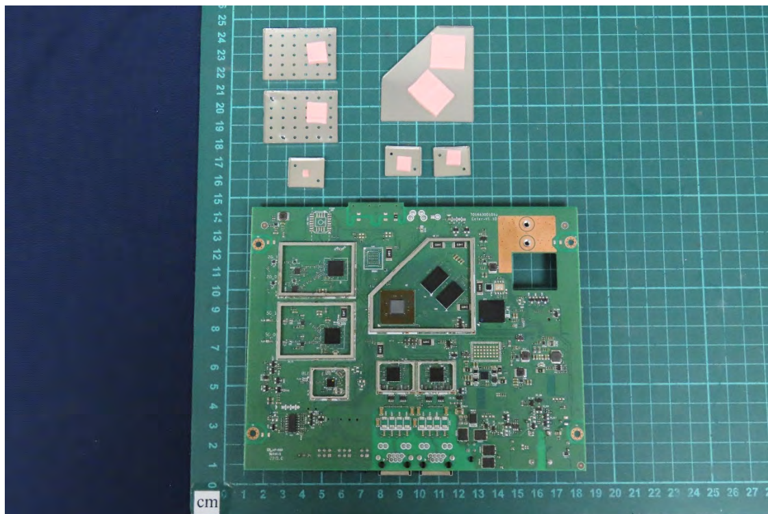
(52) EUT Photo
