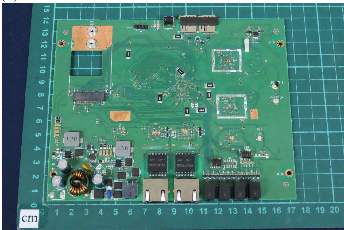
(31) EUT Photo
