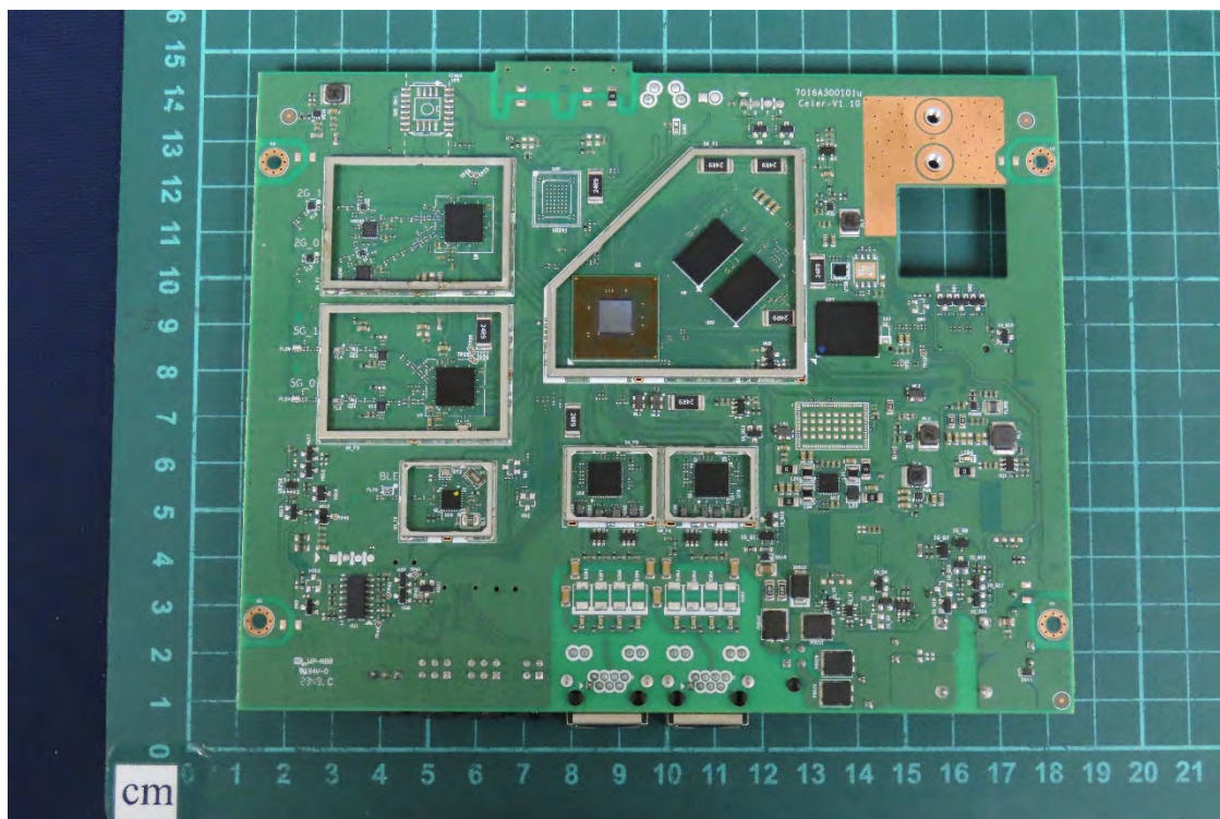
(53) EUT Photo
